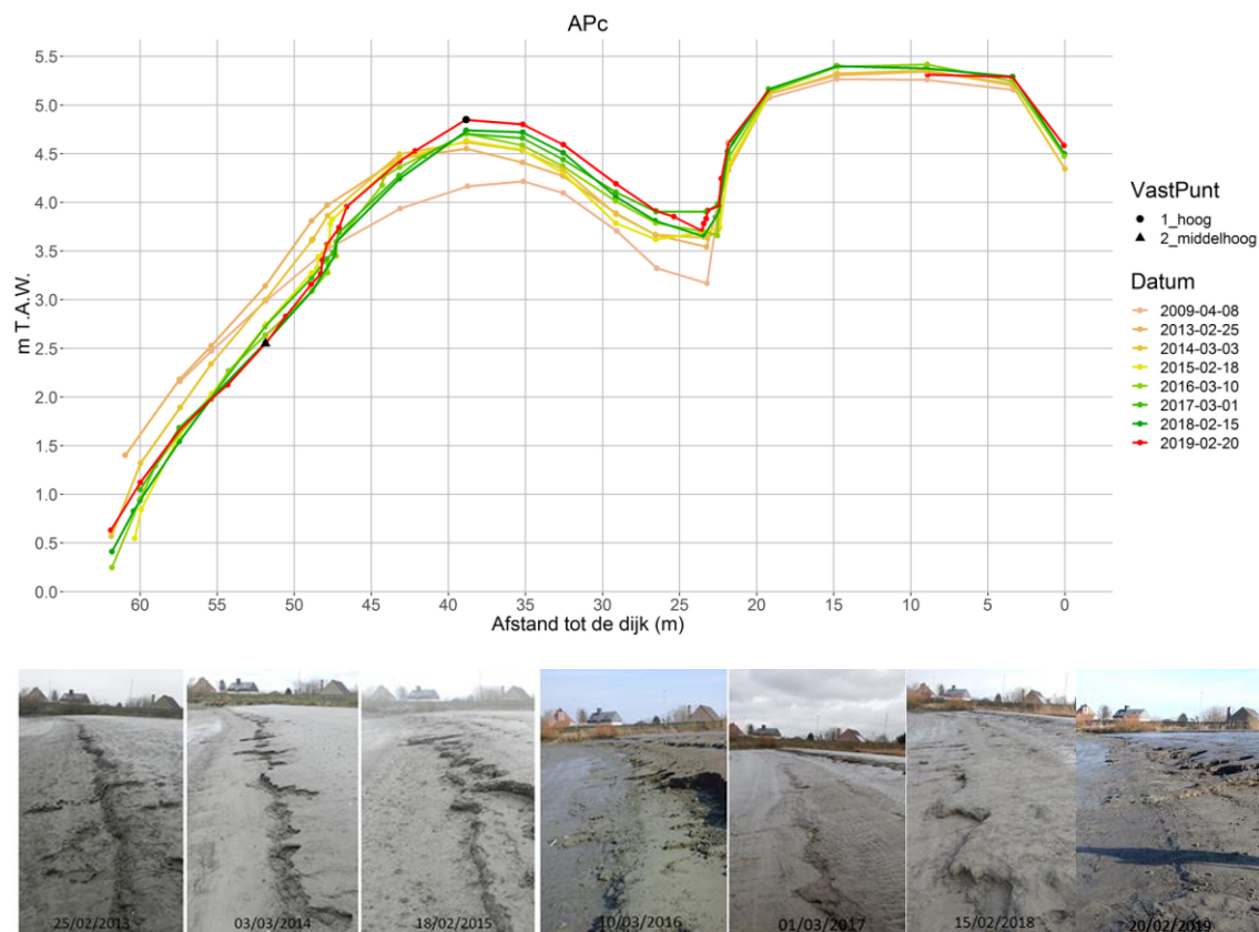
Figuur 2-3. Evolutie erosie slikklif ter hoogte van het nieuw schor van Appels.
