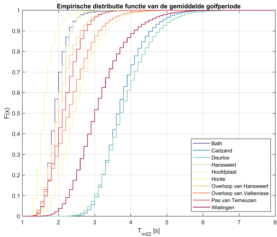
Figure 42: Empirische distributiefunctie voor de significante golfperiode berekend op basis van het spectrum voor alle beschikbare data vanaf 1998.
