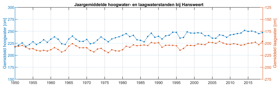
Figure 12: Jaargemiddelde hoog- en laagwaterstanden bij Hansweert
