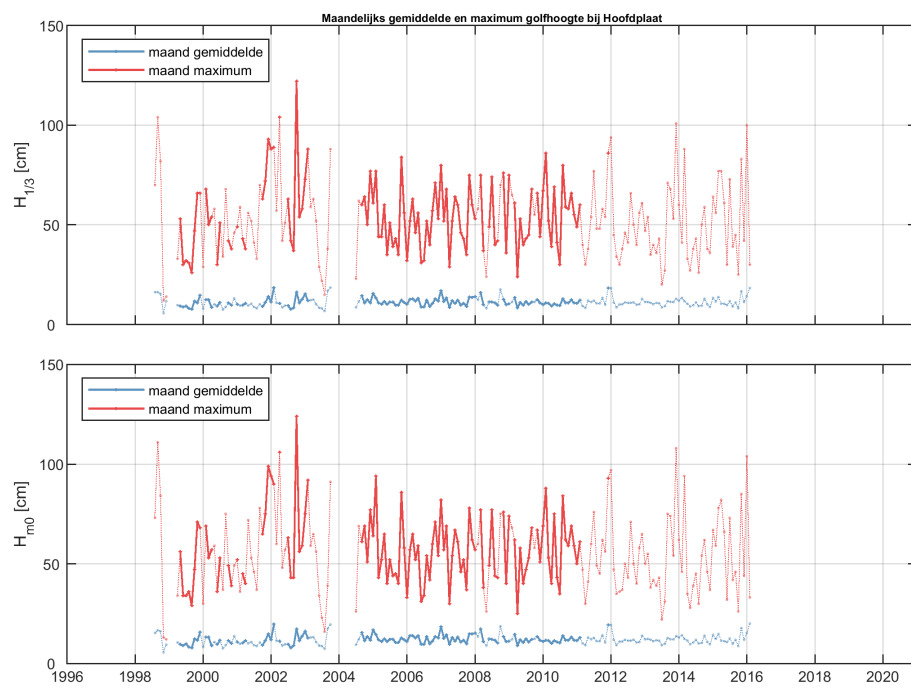
Figure 34: Maandelijks gemiddelde en maximum van de significante golfhoogte H_{1/3} (boven) en H_{m0} (onder) voor station Hoofdplaat.
