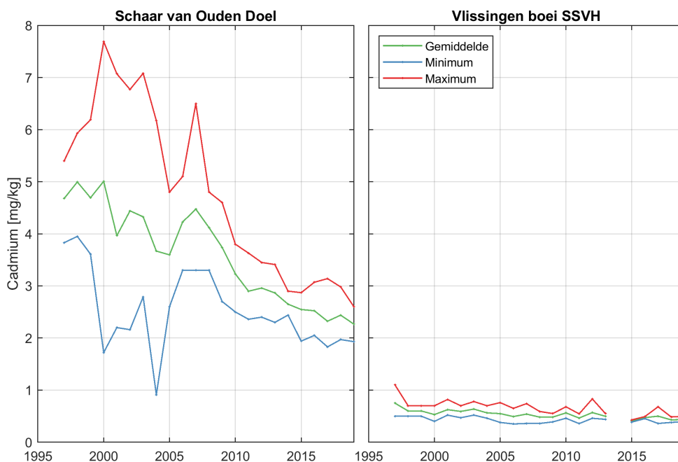
Figure 142: Jaarlijks gemiddelde (groen), minimum (blauw) en maximum (rood) van Cadmium voor beide stations.
