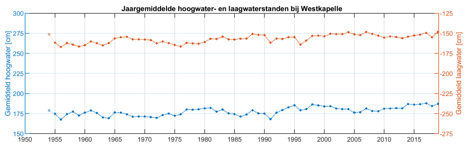
Figure 6: Jaargemiddelde hoog- en laagwaterstanden bij Westkapelle
