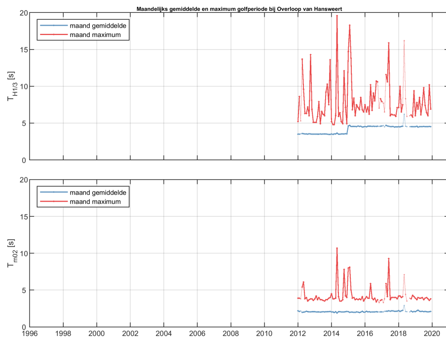
Figure 49: Maandlijks gemiddelde en maximum van de golfperiode T_{H1/3} (boven) en T_{M02} (onder) voor station Overloop van Hansweert.
