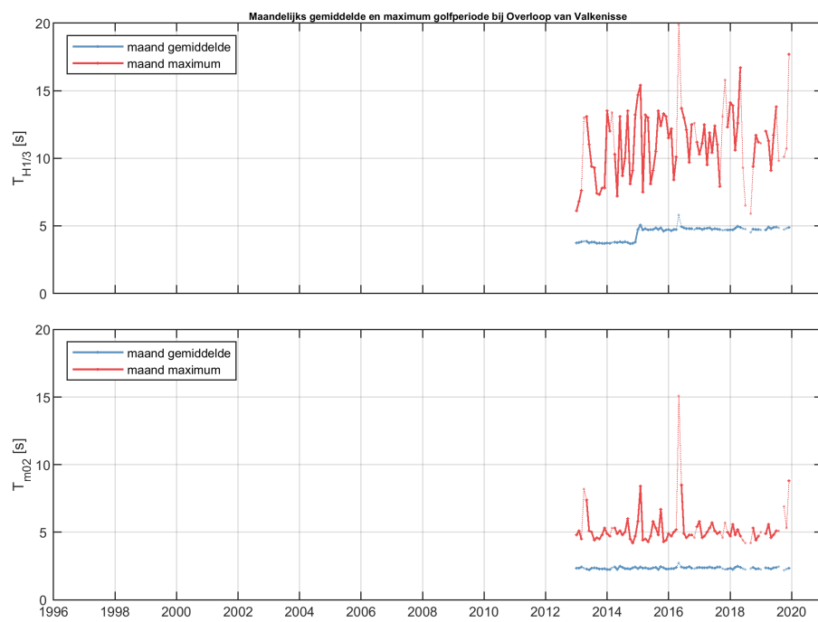
Figure 51: Maandelijks gemiddelde en maximum van de golfperiode T_{H1/3} (boven) en T_{M02} (onder) voor station Overloop van Valkenisse.
