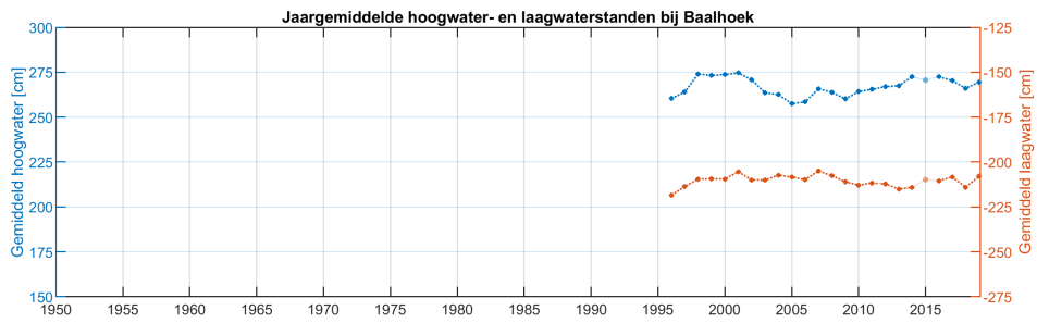
Figure 14: Jaargemiddelde hoog- en laagwaterstanden bij Baalhoek
