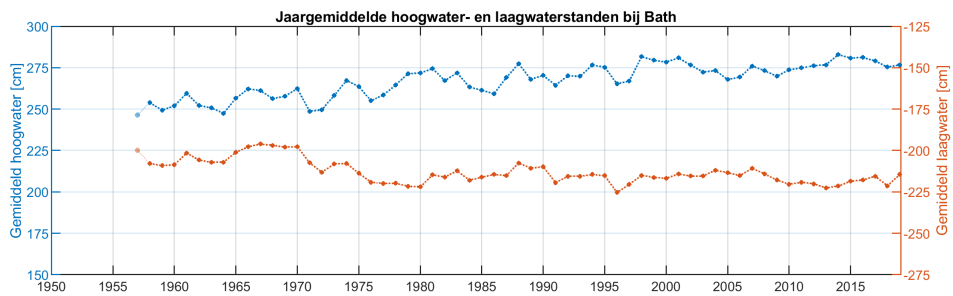
Figure 16: Jaargemiddelde hoog- en laagwaterstanden bij Bath
