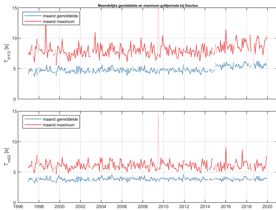
Figure 43: Maandelijks gemiddelde en maximum van de golfperiode T_{H1/3} (boven) en T_{M02} (onder) voor station Deurloo.
