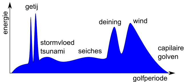
Figure 27: Voorbeeld van een geschematiseerd golfspectrum op zee (naar: www.infrawiki.nl ).
