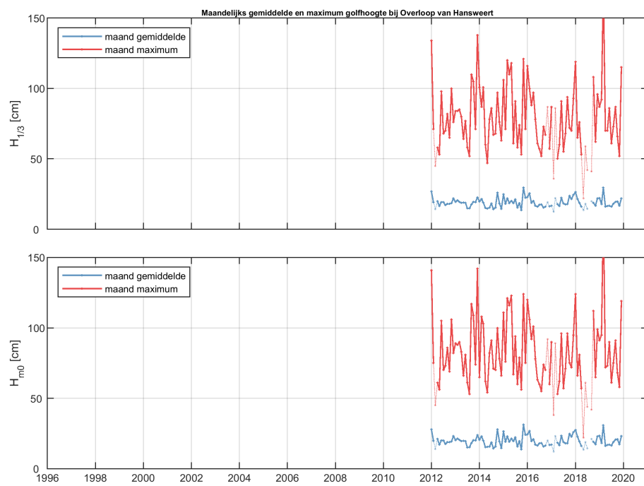
Figure 37: Maandlijks gemiddelde en maximum van de significante golfhoogte H_{1/3} (boven) en H_{m0} (onder) voor station Overloop van Hansweert.
