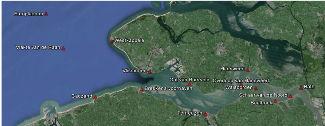
Figure 2: Ligging van de meetstations voor de waterstanden
