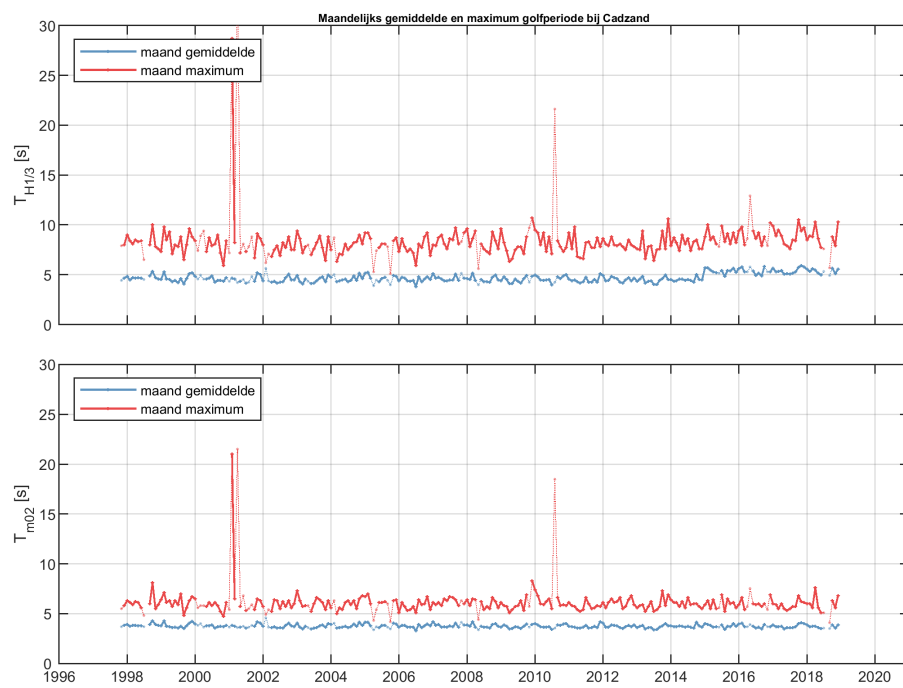
Figure 44: Maandelijks gemiddelde en maximum van de golfperiode T_{H1/3} (boven) en T_{M02} (onder) voor station Cadzand.
