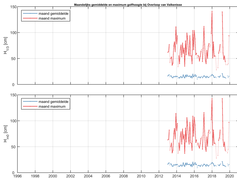
Figure 39: Maandlijks gemiddelde en maximum van de significante golfhoogte H_{1/3} (boven) en H_{m0} (onder) voor station Overloop van Valkenisse.
