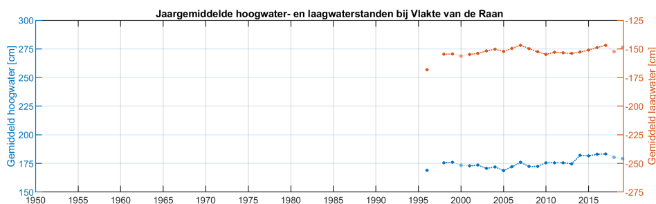
Figure 4: Jaargemiddelde hoog- en laagwaterstanden bij de Vlakte van Raan
