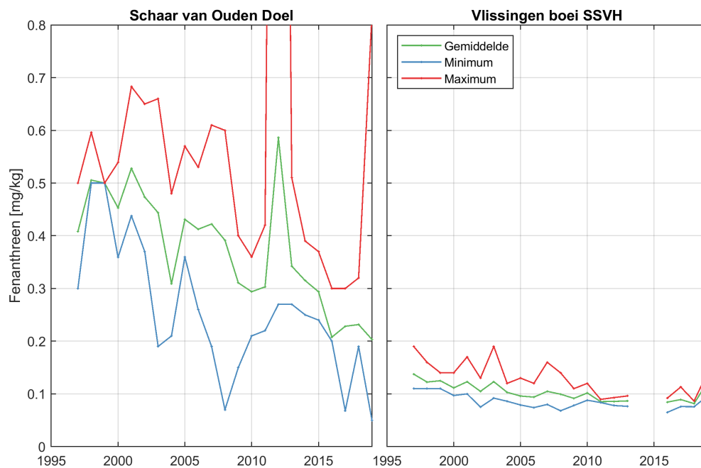
Figure 156: Jaarlijks gemiddelde (groen), minimum (blauw) en maximum (rood) van Fenanthreen voor beide stations.
