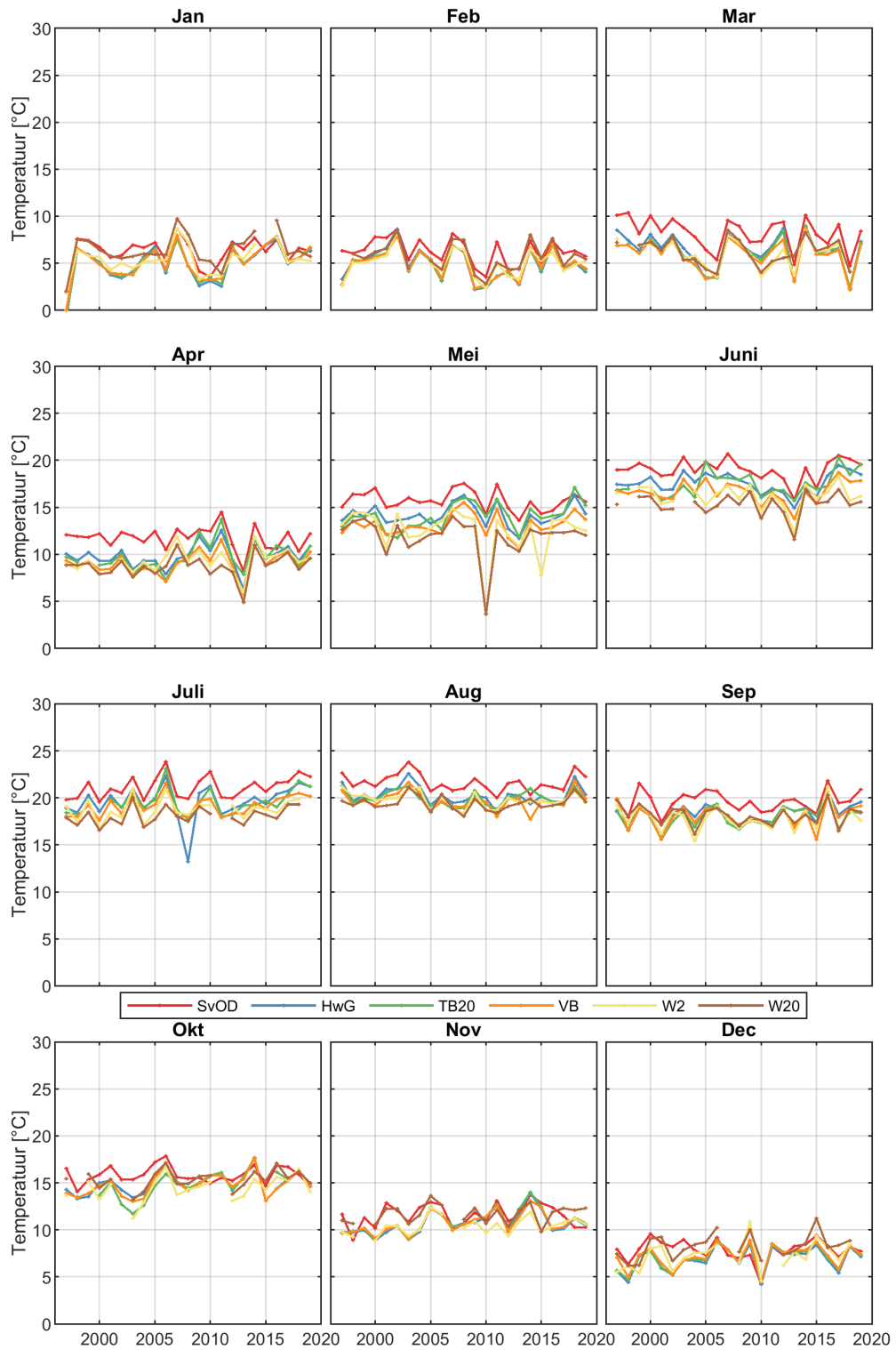
Figure 61: Maandgemiddelde temperatuur in het oppervlaktewater van de Westerschelde en de monding.
