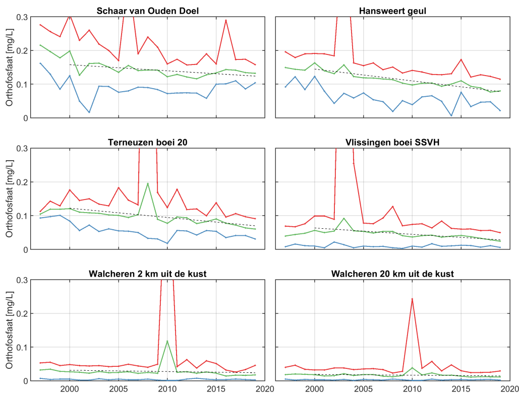
Figure 94: Jaarlijks gemiddelde, minimum en maximum van het orthofosfaatgehalte in het oppervlaktewater van de Westerschelde en de monding.
