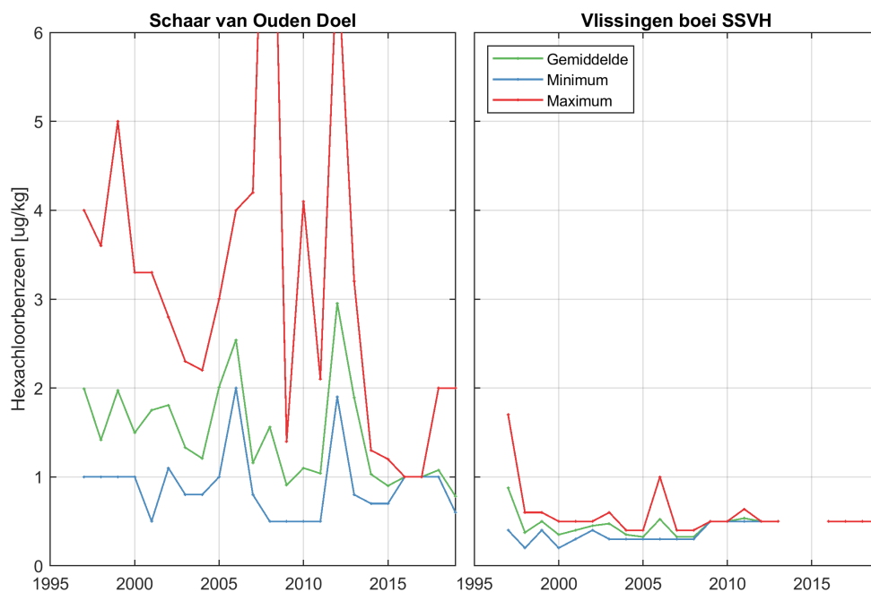
Figure 168: Jaarlijks gemiddelde (groen), minimum (blauw) en maximum (rood) van Hexachlorobenzeen voor beide stations.
