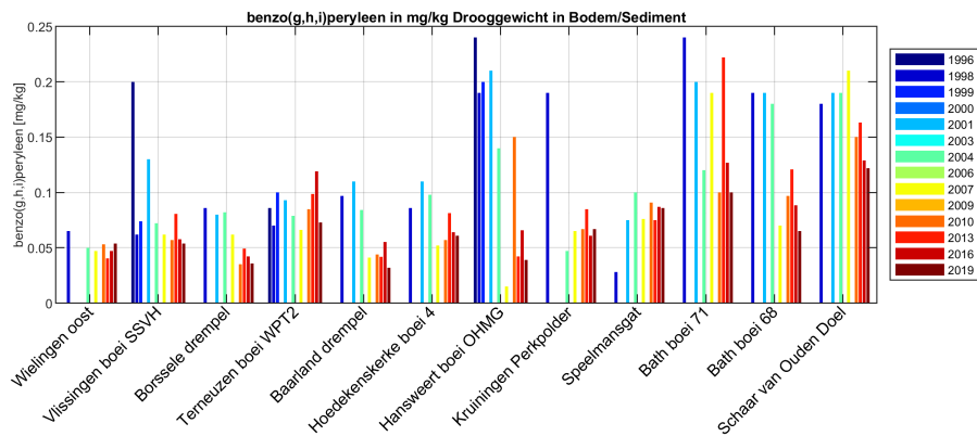
Figure 181: Benzo(g,h,i)perylene in het bodemsediment in de Westerschelde
