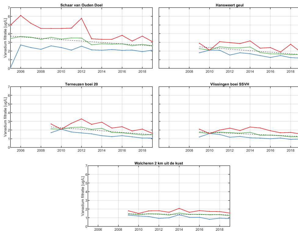
Figure 131: Jaarlijks gemiddelde, minimum en maximum van het gefilterde vanadiumgehalte in het oppervlaktewater van de Westerschelde en de monding.
