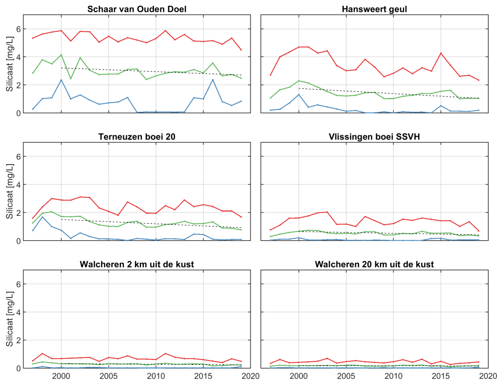
Figure 101: Jaarlijks gemiddelde, minimum en maximum van het silicaatgehalte in het oppervlaktewater van de Westerschelde en de monding.
