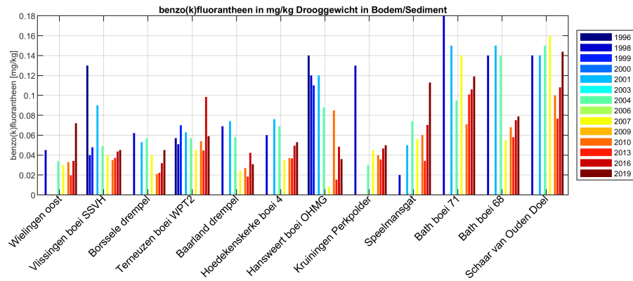
Figure 182: Benzo(k)fluorantheen in het bodemsediment in de Westerschelde
