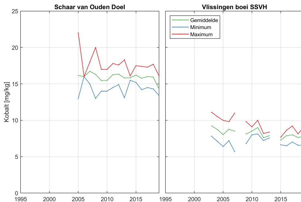
Figure 144: Jaarlijks gemiddelde (groen), minimum (blauw) en maximum (rood) van Kobalt voor beide stations.
