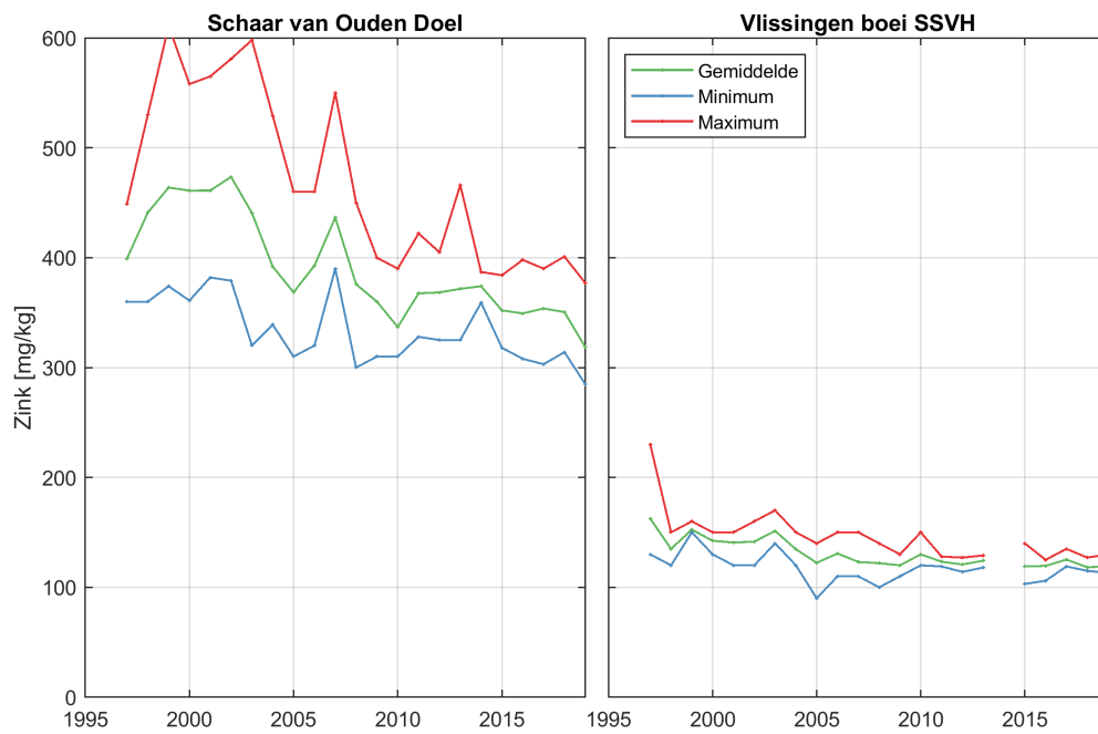
Figure 149: Jaarlijks gemiddelde (groen), minimum (blauw) en maximum (rood) van Zink voor beide stations.
