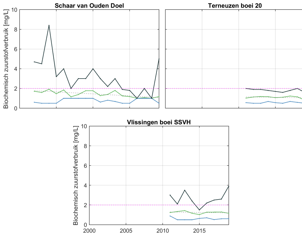
Figure 76: Jaarlijks gemiddelde, minimum en maximum van het biochemisch zuurstofverbruik in het oppervlaktewater van de Westerschelde en de monding. De roze stippellijn is de bepalingsgrens.
