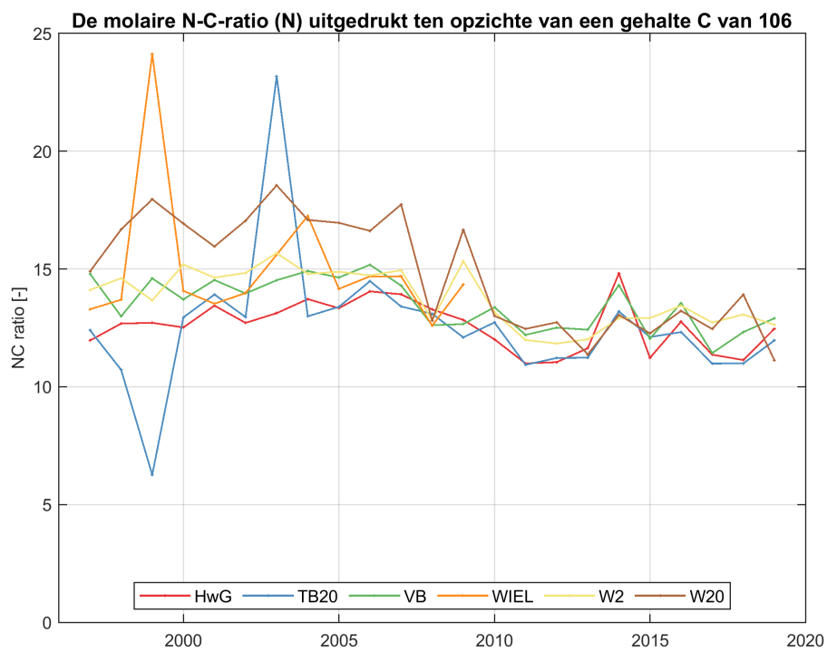
Figure 108: De molaire N-C-ratio, N uitgedrukt ten opzichte van een gehalte C van 106, gemiddeld over een jaar in het oppervlaktewater van de Westerschelde en de monding.
