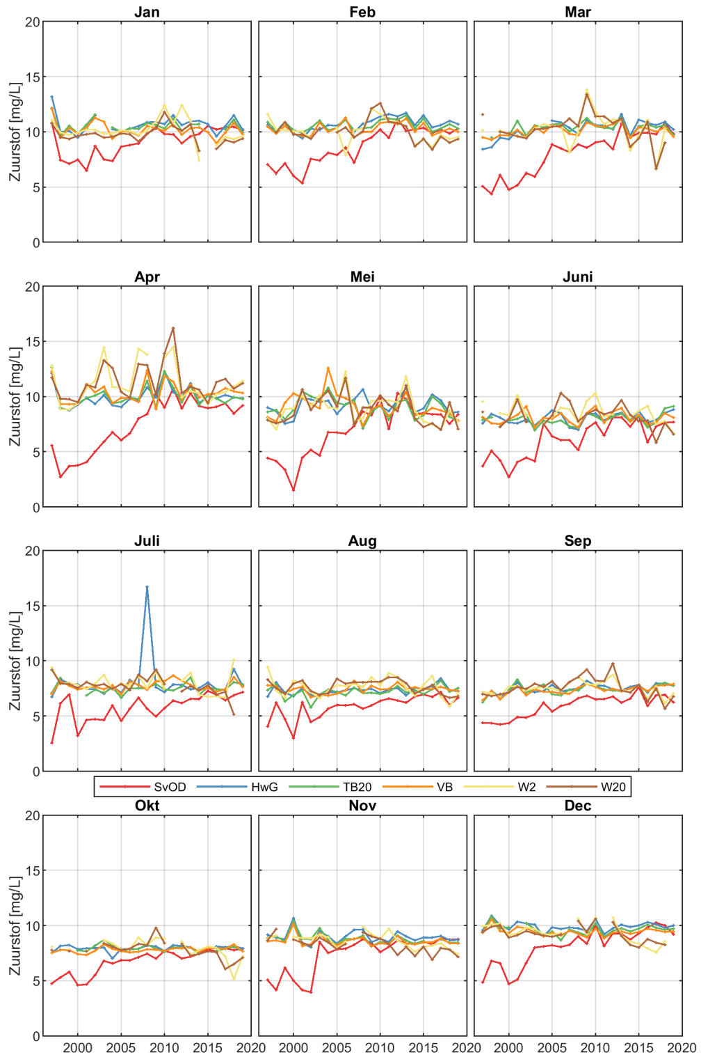
Figure 66: Maandgemiddelde zuurstofgehalten in mg/L in het oppervlaktewater van de Westerschelde en de monding.
