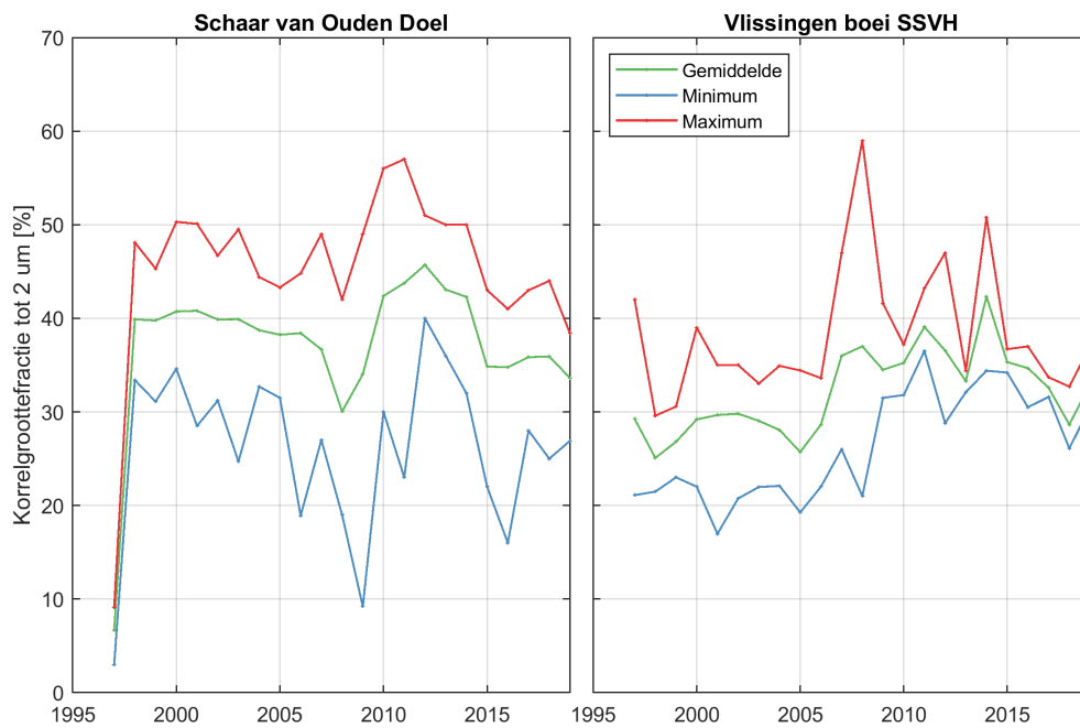
Figure 140: Jaarlijks gemiddelde (groen), minimum (blauw) en maximum (rood) van de korrelgroottefractie tot 2\mu\text{m} voor beide stations
