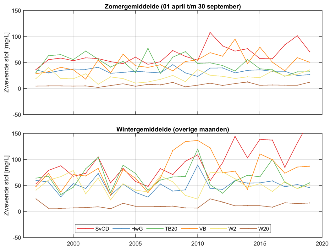
Figure 84: Gemiddeld waarden voor de hoeveelheid zwevende stof gedurende de zomer en de winter in het oppervlaktewater van de Westerschelde en de monding.
