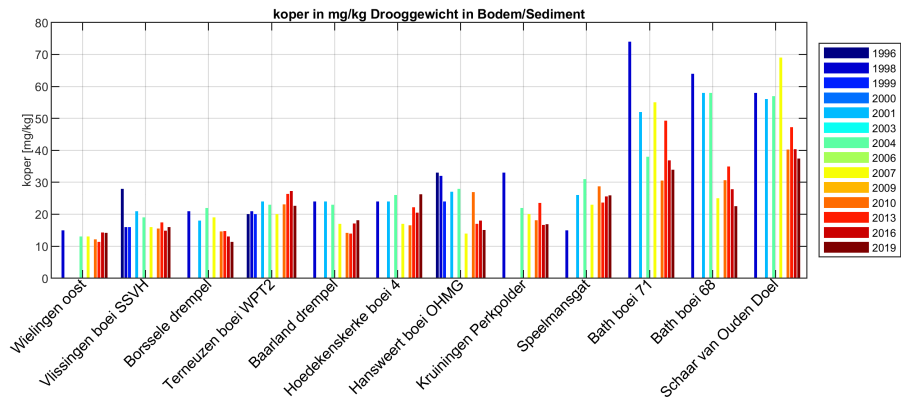
Figure 174: Koper in het bodemsediment in de Westerschelde
