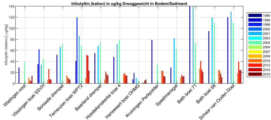
Figure 195: Tributyltin in het bodemsediment in de Westerschelde
