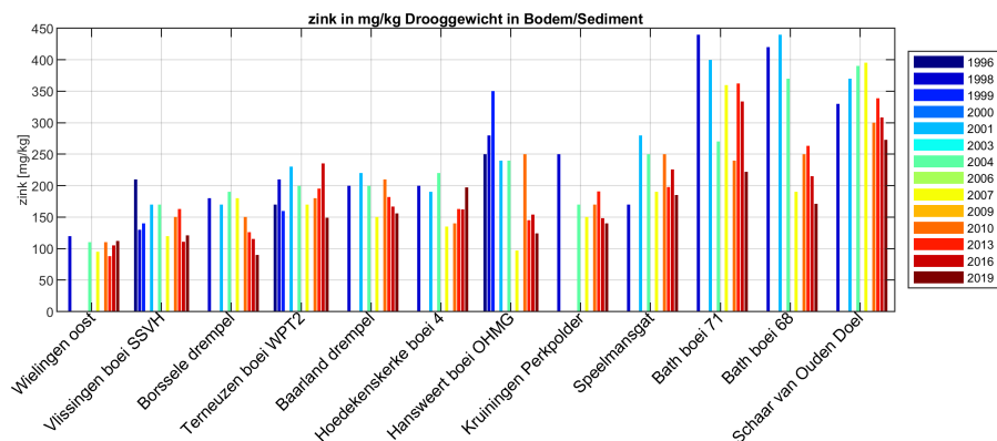
Figure 177: Zink in het bodemsediment in de Westerschelde
