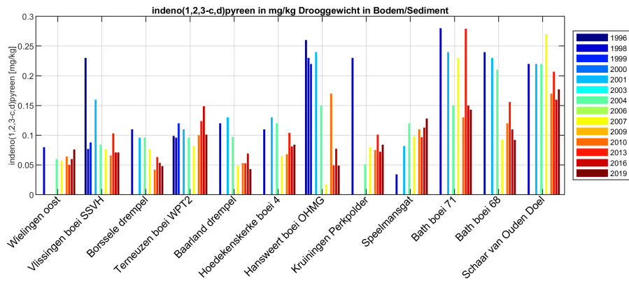
Figure 186: Indeno(1,2,3-c,d)pyreen in het bodemsediment in de Westerschelde
