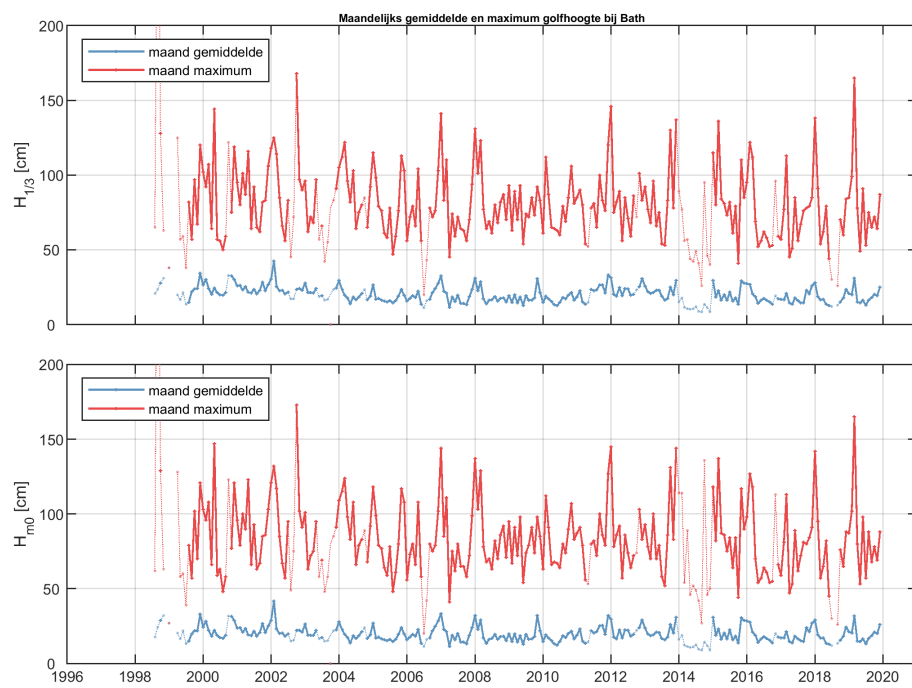
Figure 40: Maandelijks gemiddelde en maximum van de significante golfhoogte H_{1/3} (boven) en H_{m0} (onder) voor station Bath.
