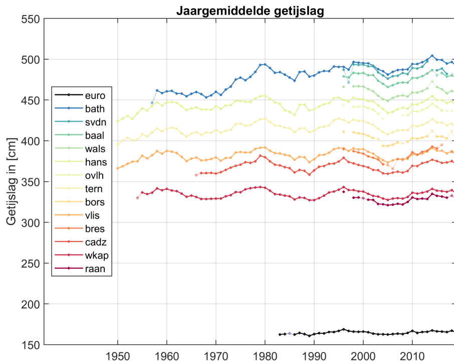
Figure 19: De gemiddelde getijslag over tijd op de Noordzee, in de monding en in de Westerschelde. Dunnere en transparante kleuren geven jaarlijkse gemiddeldes aan met twee of meer maanden met missende data.
