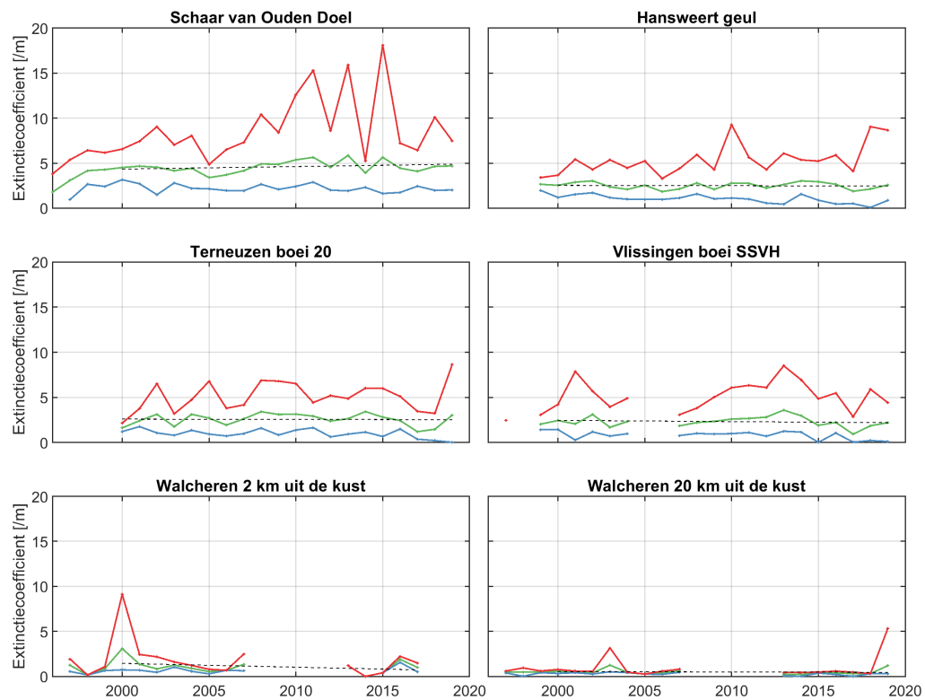
Figure 79: Jaarlijks gemiddelde, minimum en maximum van de extinctiecoëfficiënt in het oppervlaktewater van de Westerschelde en de monding.
