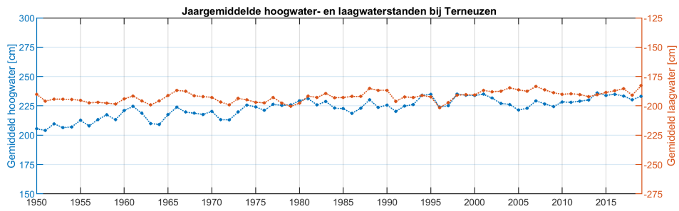
Figure 11: Jaargemiddelde hoog- en laagwaterstanden bij Terneuzen
