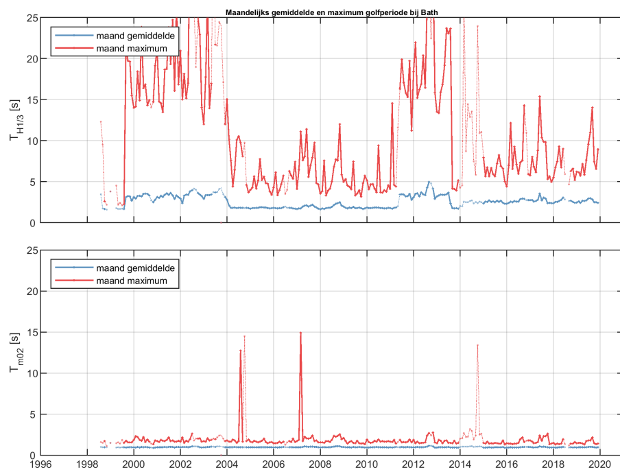
Figure 52: Maandelijks gemiddelde en maximum van de golfperiode T_{H1/3} (boven) en T_{M02} (onder) voor station Bath.
