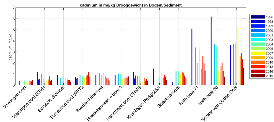
Figure 172: Cadmium in het bodemsediment in de Westerschelde
