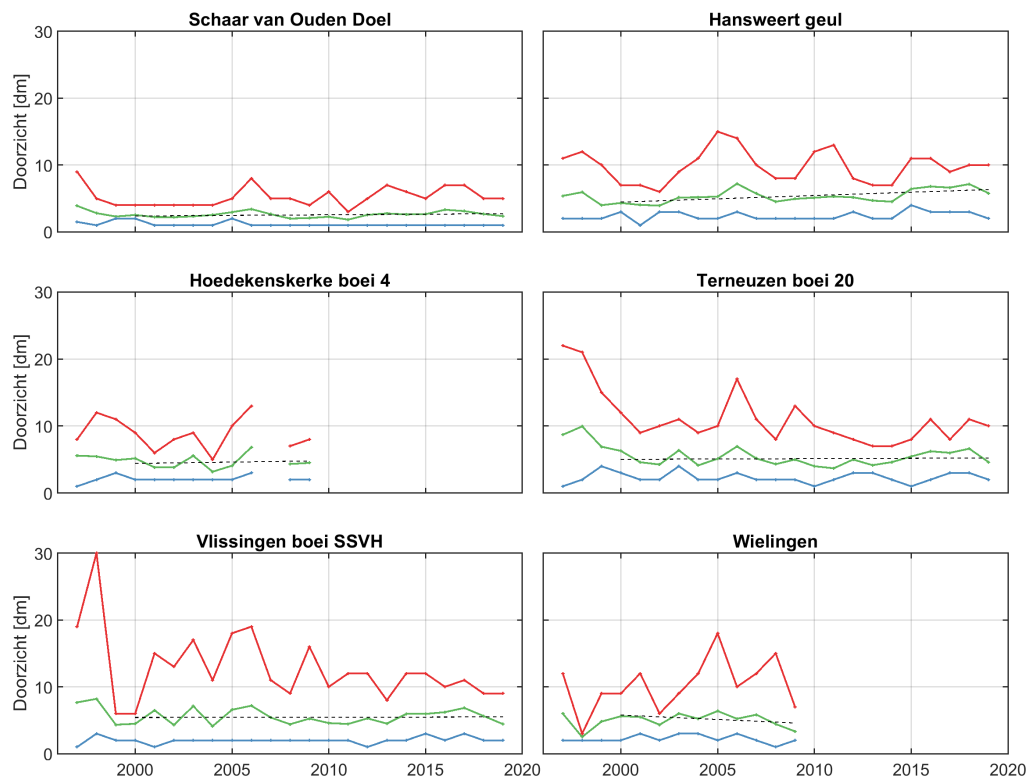
Figure 78: Jaarlijks gemiddelde, minimum en maximum van het doorzicht in het oppervlaktewater van de Westerschelde en de monding.
