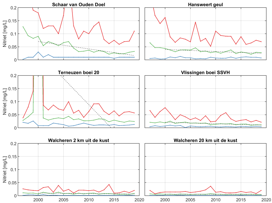
Figure 90: Jaarlijks gemiddelde, minimum en maximum van het nitrietgehalte in het oppervlaktewater van de Westerschelde en de monding.
