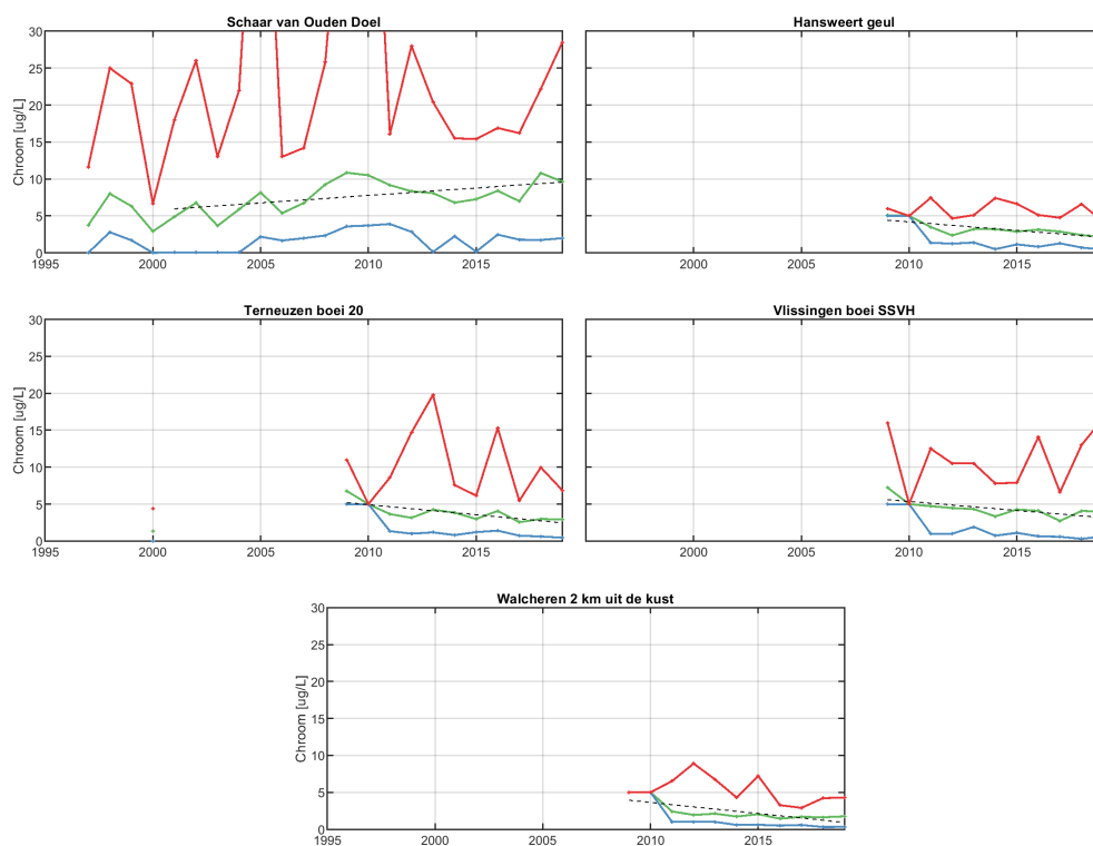
Figure 118: Jaarlijks gemiddelde, minimum en maximum van het totale chroomgehalte in het oppervlaktewater van de Westerschelde en de monding
