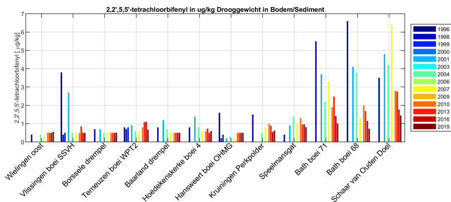
Figure 191: PCB52 in het bodemsediment in de Westerschelde
