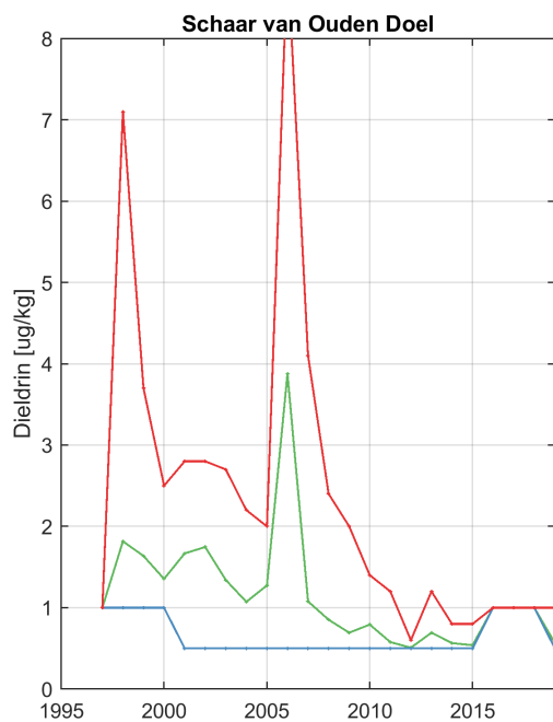
Figure 167: Jaarlijks gemiddelde (groen), minimum (blauw) en maximum (rood) van Dieldrin voor beide stations.
