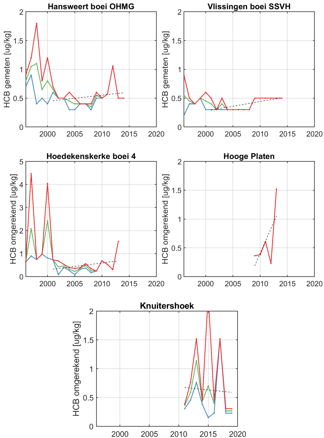
Figure 222: Jaarlijks gemiddelde (groen), minimum (blauw) en maximum (rood) voor het gehalte hexachloorbenzeen in mosselen (nat en droog) voor meerdere stations. Waardes zijn in drooggewicht gepresenteerd.
