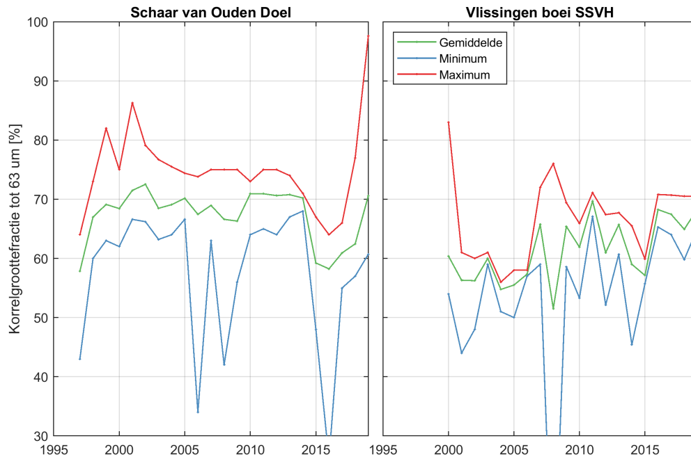
Figure 139: Jaarlijks gemiddelde (groen), minimum (blauw) en maximum (rood) van de korrelgroottefractie tot 63\mu\text{m} voor 2 stations
