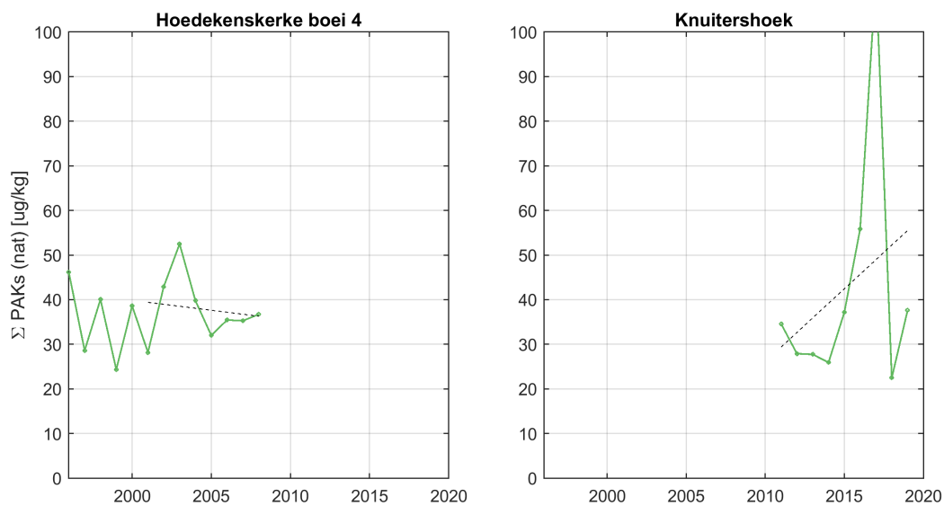
Figure 217: Jaarlijks gesommeerde waarde van de 6 PAK's van Borneff in mossel bij Hoedekenskerke boei 4 en Knuitershoek. Waardes zijn in natgewicht gepresenteerd.
