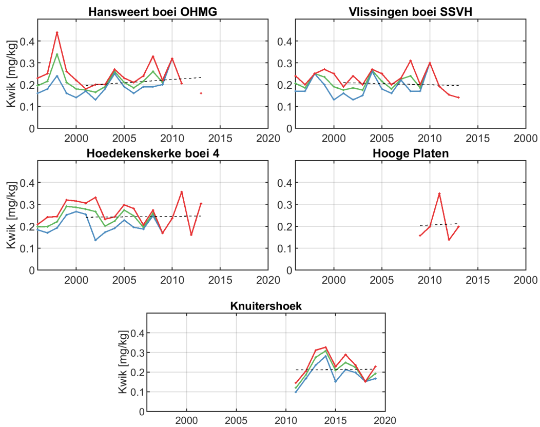
Figure 209: Jaarlijks gemiddelde (groen), minimum (blauw) en maximum (rood) voor kwik in mosselen (nat en droog) voor meerdere stations. Waardes zijn in drooggewicht gepresenteerd.
