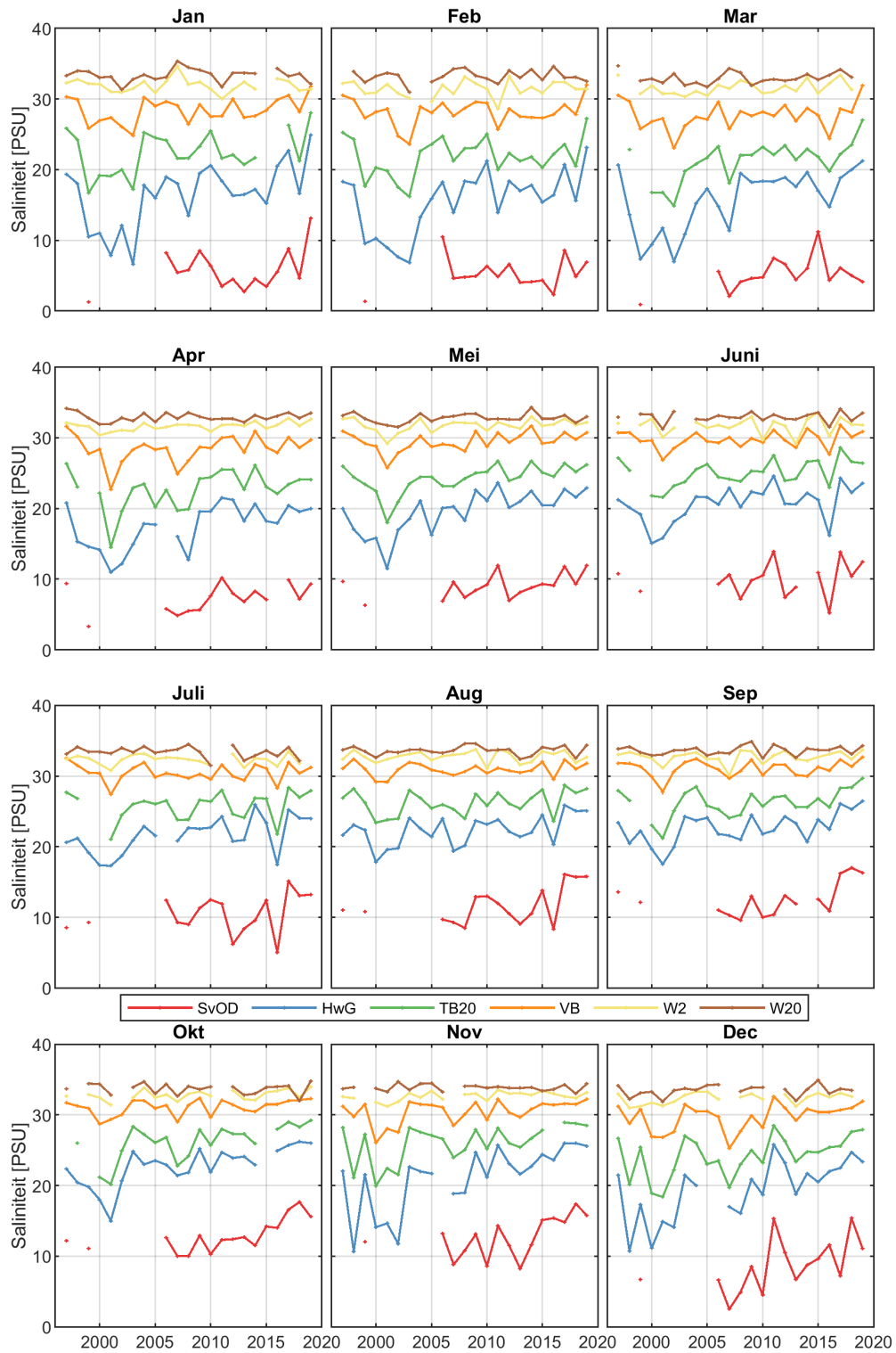
Figure 57: Maandgemiddelde saliniteit in het oppervlaktewater van de Westerschelde en de monding.
