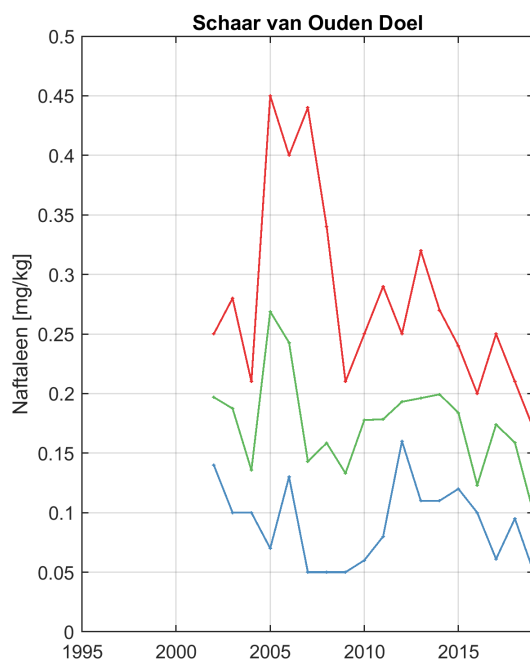
Figure 159: Jaarlijks gemiddelde (groen), minimum (blauw) en maximum (rood) van Naftaleen voor beide stations.
