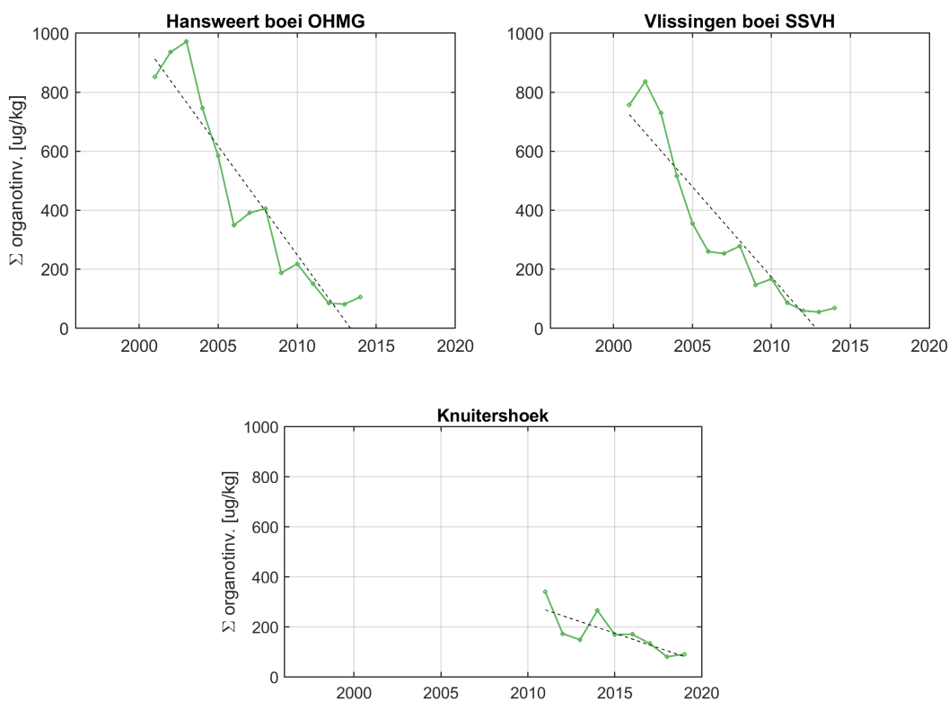
Figure 221: Jaarlijks gesommeerde waarde van de organotinverbindingen in mossel voor 3 stations in de Westerschelde. Waardes zijn in drooggewicht gepresenteerd.
