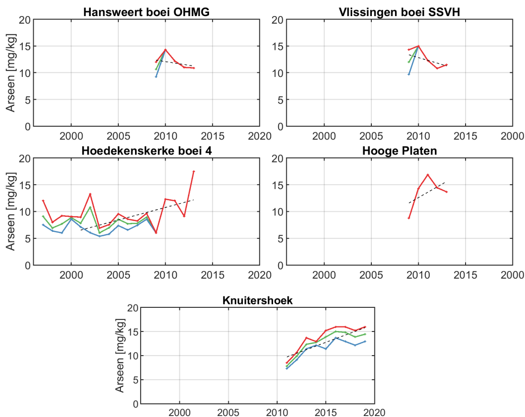
Figure 201: Jaarlijks gemiddelde (groen), minimum (blauw) en maximum (rood) voor arseen in mosselen (nat en droog) voor meerdere stations. Waardes zijn in drooggewicht gepresenteerd.
