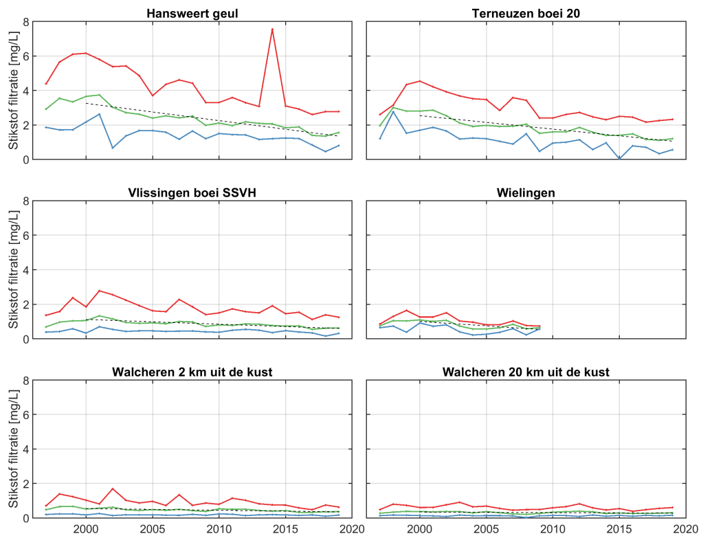
Figure 85: Jaarlijks gemiddelde, minimum en maximum van het stikstofgehalte in het oppervlaktewater van de Westerschelde en de monding.
