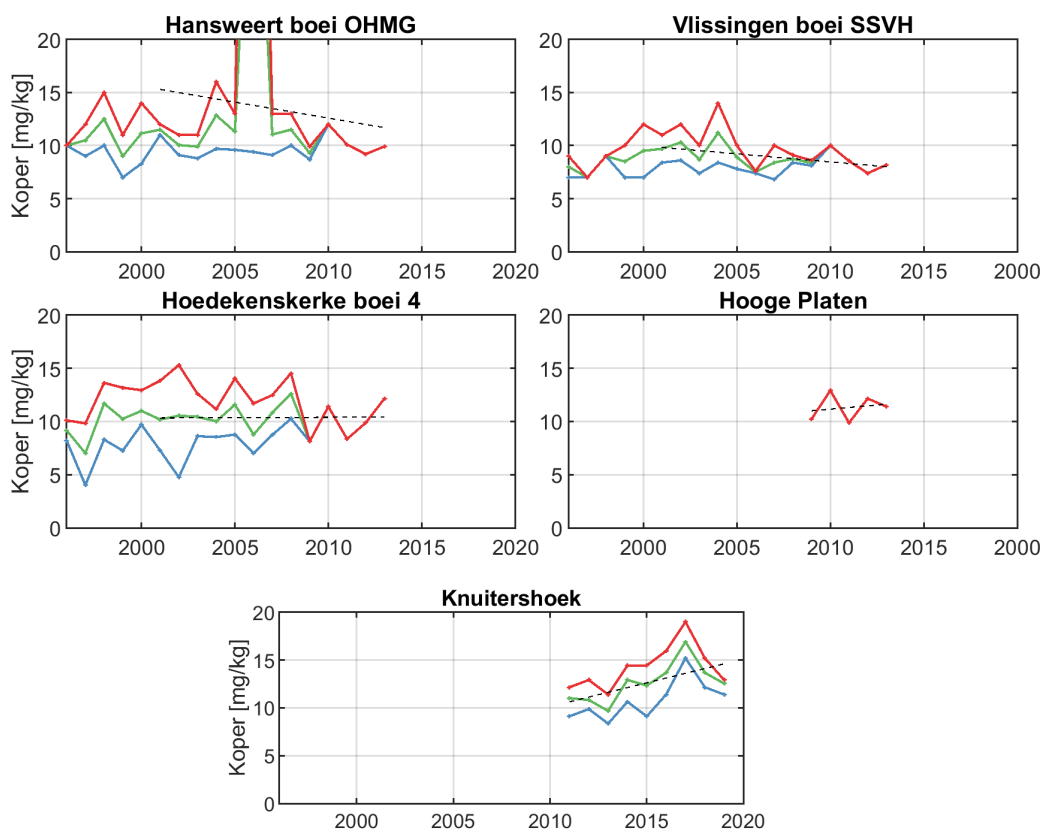
Figure 206: Jaarlijks gemiddelde (groen), minimum (blauw) en maximum (rood) voor koper in mosselen (nat en droog) voor meerdere stations. Waardes zijn in drooggewicht gepresenteerd.
