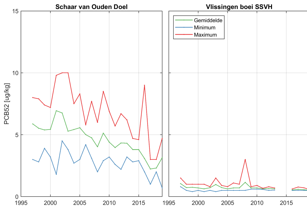
Figure 164: Jaarlijks gemiddelde (groen), minimum (blauw) en maximum (rood) van PCB52 voor beide stations.
