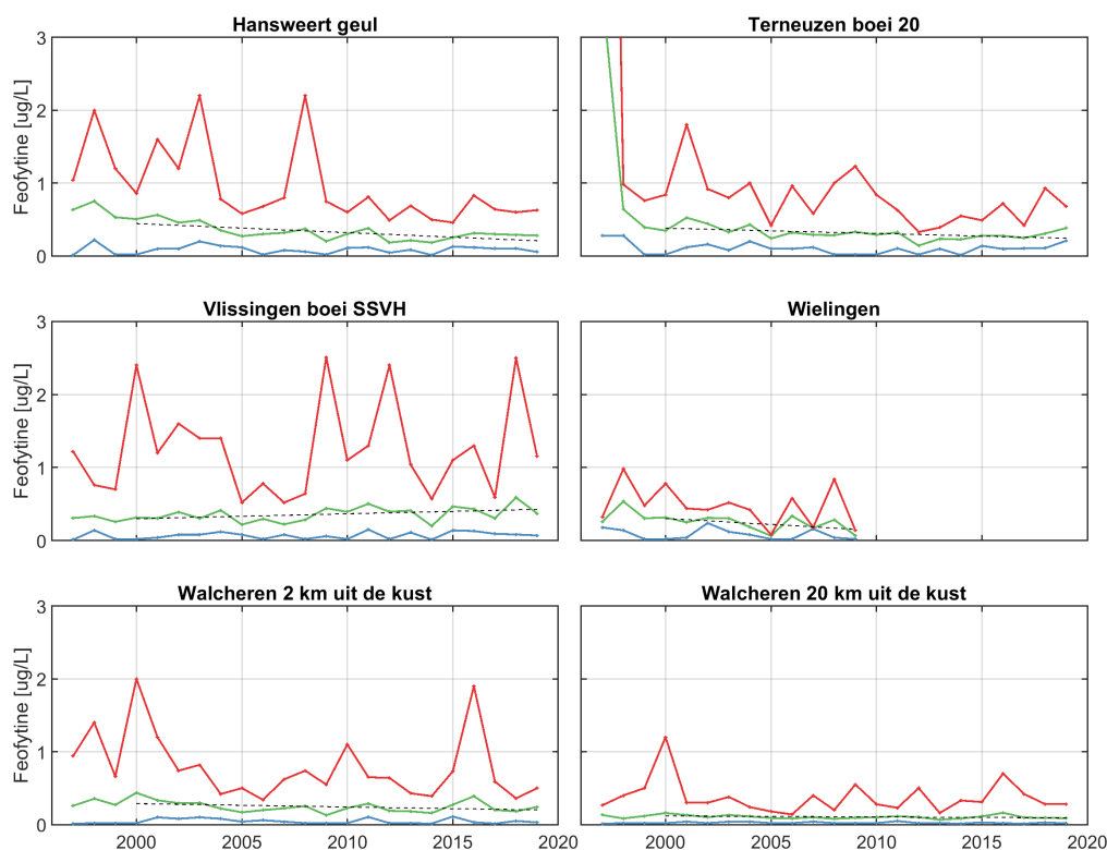
Figure 70: Jaarlijks gemiddelde, minimum en maximum van feofytine in het oppervlaktewater van de Westerschelde en de monding.
