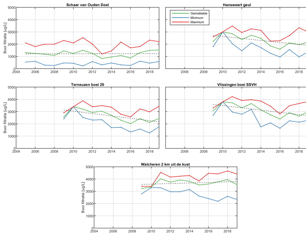
Figure 115: Jaarlijks gemiddelde, minimum en maximum van het gefilterde boorgehalte in het oppervlakte-water van de Westerschelde en de monding
