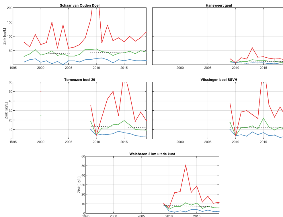
Figure 134: Jaarlijks gemiddelde, minimum en maximum van het totale zinkgehalte in het oppervlaktewater van de Westerschelde en de monding.
