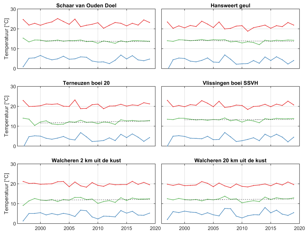
Figure 58: Jaarlijks gemiddelde (groen), minimum (blauw) en maximum (rood) van de temperatuur in de Westerschelde en in de monding vanaf 1997. In 2015 zijn er bij Walcheren alleen metingen gedaan tussen september en december, hierdoor zijn de gemiddeldes lager dan in andere jaren.
