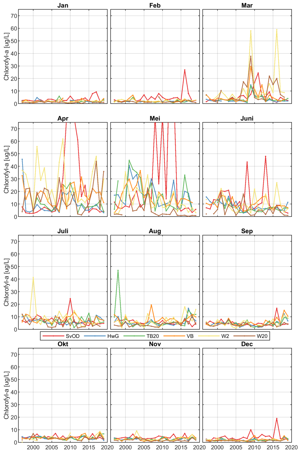
Figure 69: Maandgemiddelde chlorofyl-a in het oppervlaktewater van de Westerschelde en de monding.
