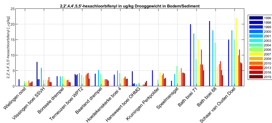
Figure 189: PCB153 in het bodemsediment in de Westerschelde
