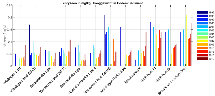
Figure 183: Chryseen in het bodemsediment in de Westerschelde
