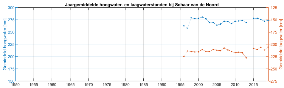
Figure 15: Jaargemiddelde hoog- en laagwaterstanden bij Schaar van de Noord
