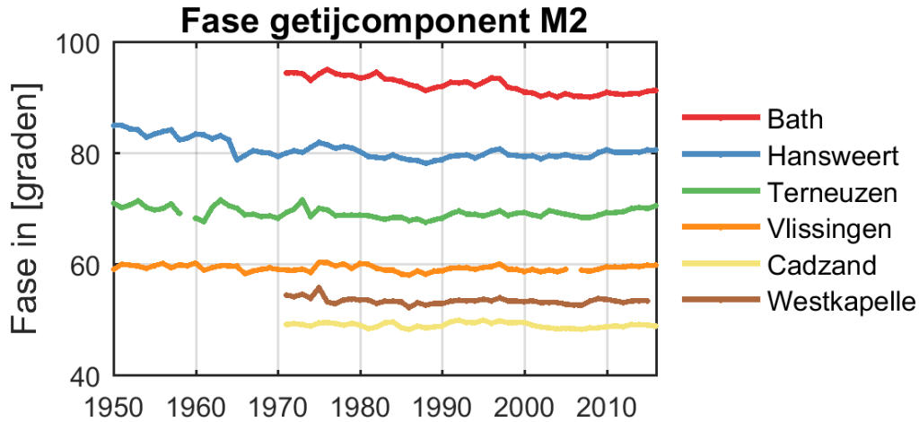
Figuur 2.24: Fase van de M2-getijcomponent voor de landelijke meetstations.
