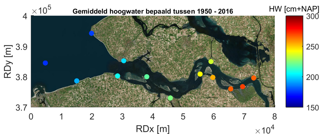
Figuur 2.18: Gemiddeld hoogwater per station berekend op alle beschikbare data tussen 1950 en 2016
