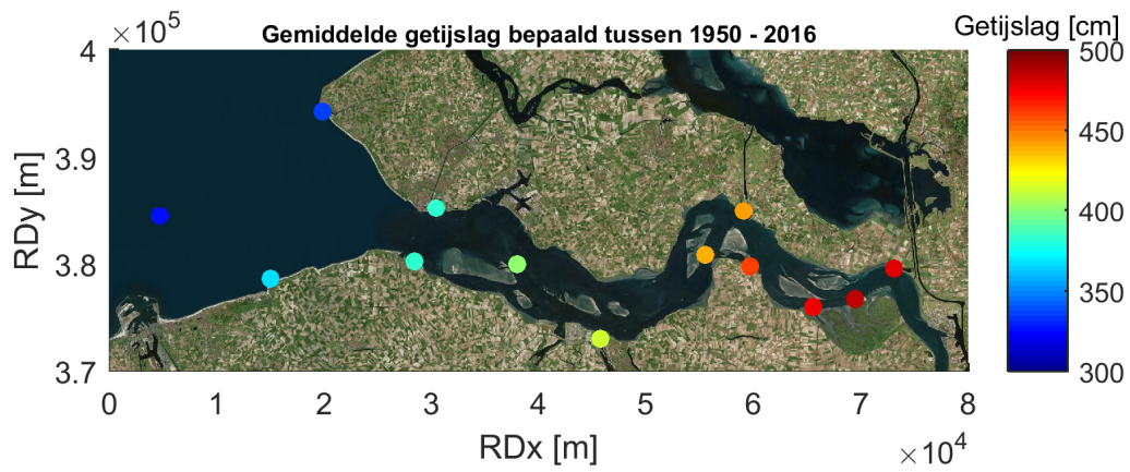
Figuur 2.20: Gemiddelde getijslag per station berekend op alle beschikbare data tussen 1950 en 2016
