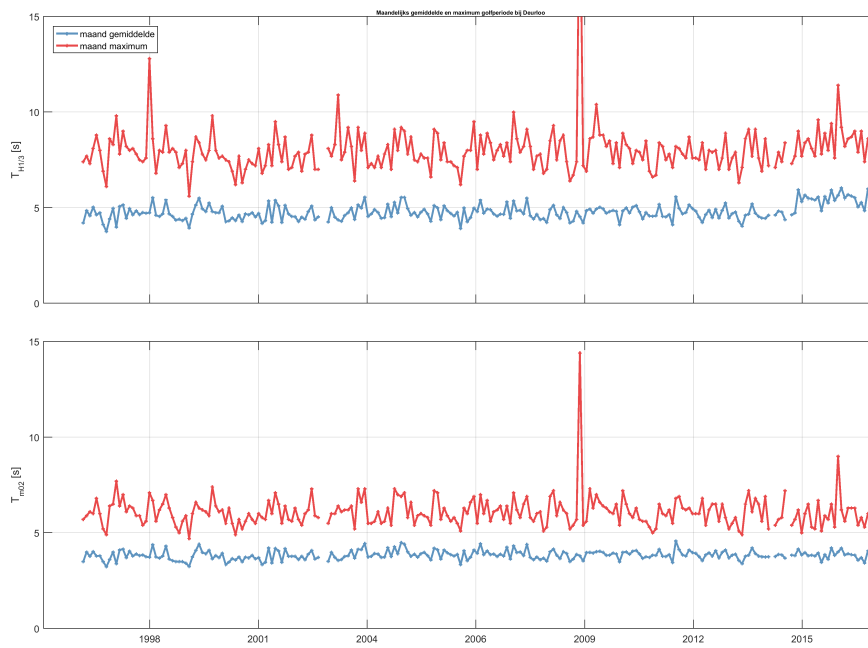
Figuur 2.42: Maandelijks gemiddelde en maximum van de golfperiode T_{H1/3} (boven) en T_{M02} (onder) voor station Deurloo.
