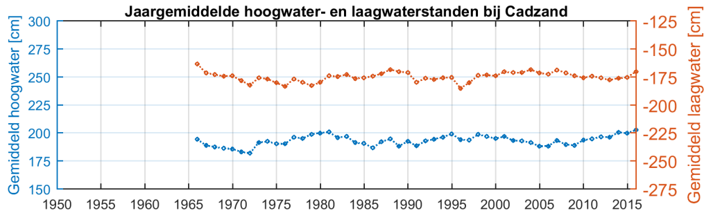
Figuur 2.5: Jaargemiddelde hoog- en laagwaterstanden bij Cadzand
