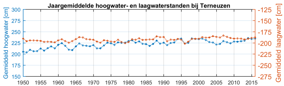
Figuur 2.11: Jaargemiddelde hoog- en laagwaterstanden bij Terneuzen
