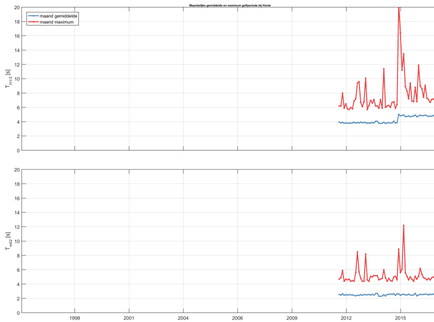
Figuur 2.46: Maandelijks gemiddelde en maximum van de golfperiode T_{H1/3} (boven) en T_{M02} (onder) voor station Honte.
