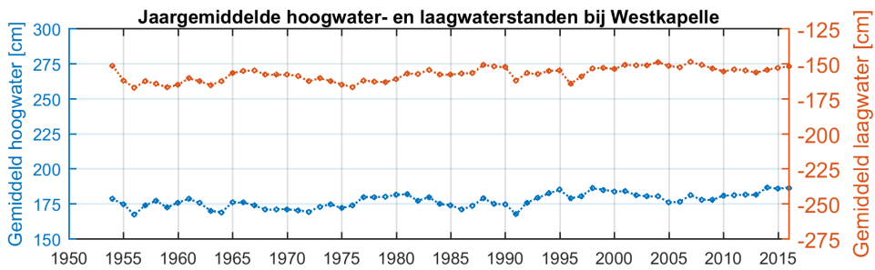
Figuur 2.6: Jaargemiddelde hoog- en laagwaterstanden bij Westkappele
