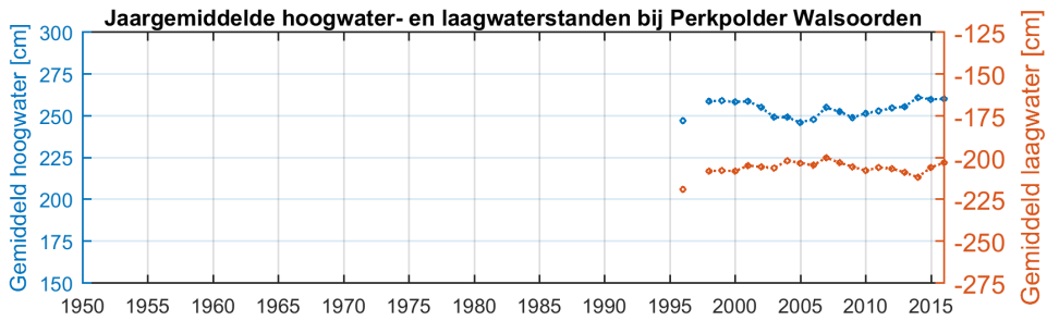
Figuur 2.13: Jaargemiddelde hoog- en laagwaterstanden bij Walsoorden
