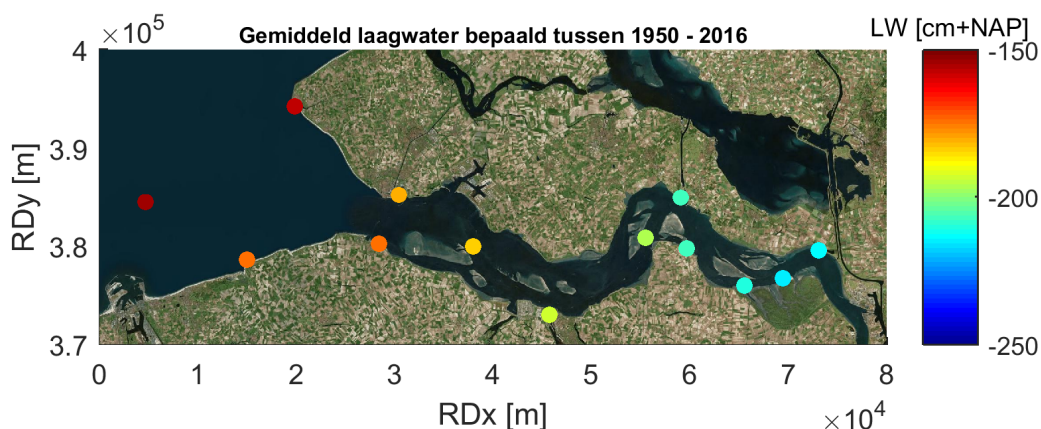
Figuur 2.17: Gemiddeld laagwater per station berekend op alle beschikbare data tussen 1950 en 2016
