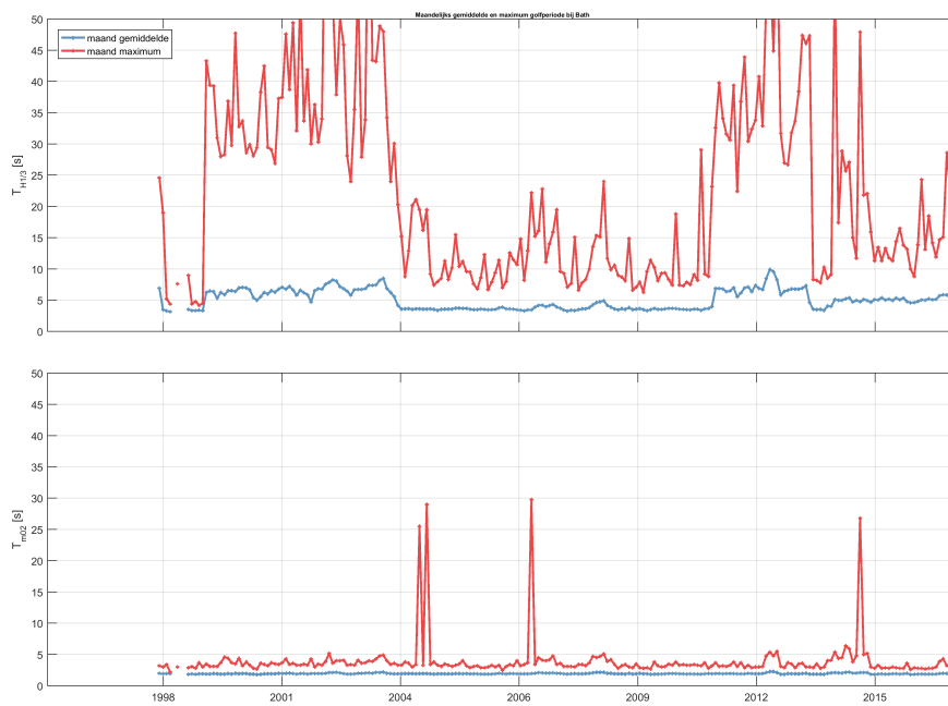
Figuur 2.50: Maandelijks gemiddelde en maximum van de golfperiode T_{H1/3} (boven) en T_{M02} (onder) voor station Bath.
