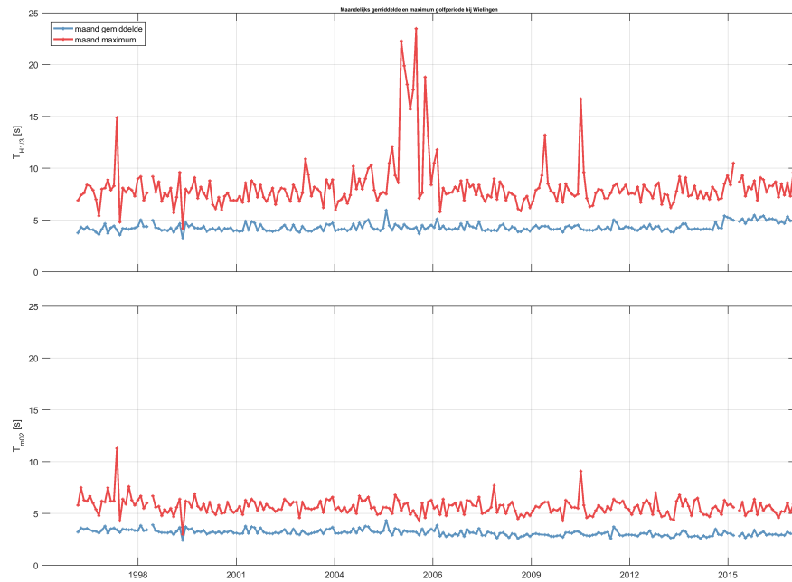
Figuur 2.44: Maandelijks gemiddelde en maximum van de golfperiode T_{H1/3} (boven) en T_{M02} (onder) voor station Wielingen.
