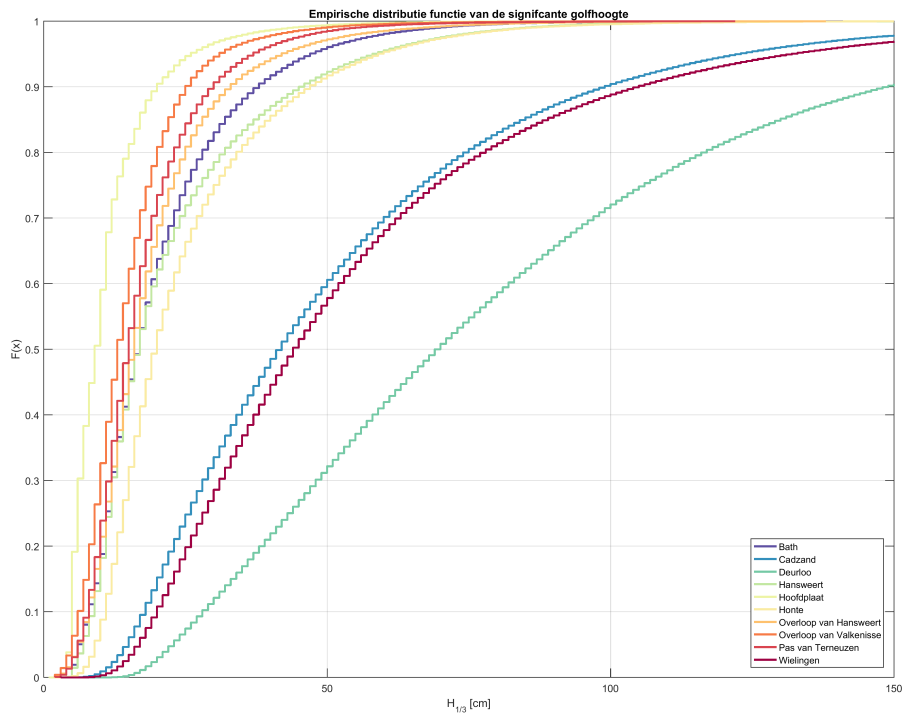
Figuur 2.30: Empirische distributiefunctie voor de significante golfhoogte berekend op basis van het spectrum voor alle beschikbare data tussen 1998 en 2015
