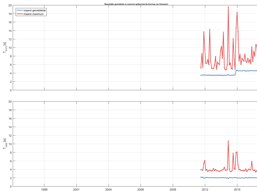
Figuur 2.47: Maandelijks gemiddelde en maximum van de golfperiode T_{H1/3} (boven) en T_{M02} (onder) voor station Overloop van Hansweert.
