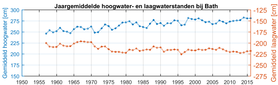
Figuur 2.16: Jaargemiddelde hoog- en laagwaterstanden bij Bath
