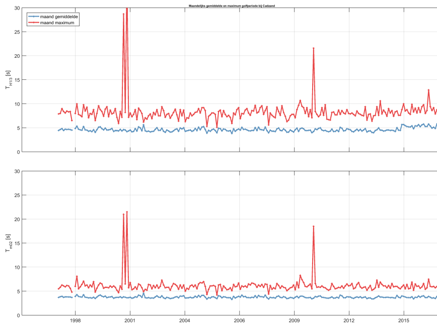
Figuur 2.43: Maandelijks gemiddelde en maximum van de golfperiode T_{H1/3} (boven) en T_{M02} (onder) voor station Cadzand.
