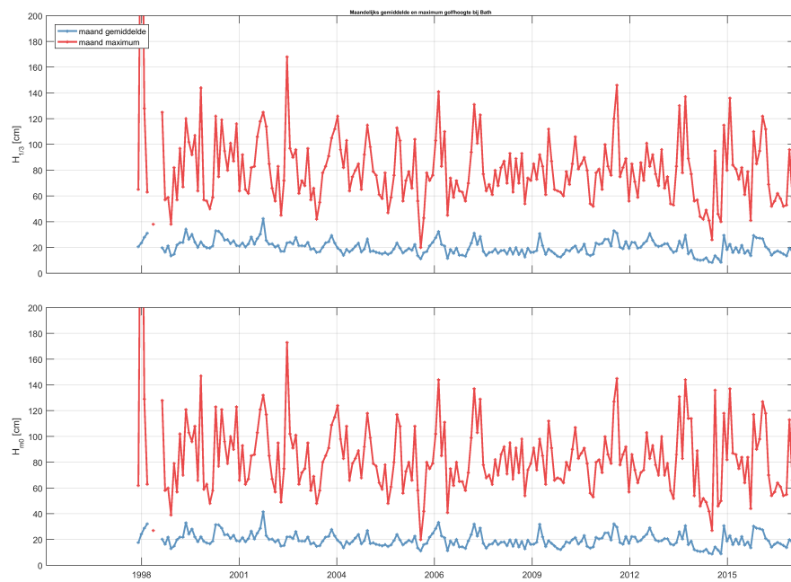
Figuur 2.39: Maandelijks gemiddelde en maximum van de significante golfhoogte H_{1/3} (boven) en H_{m0} (onder) voor station Bath.
