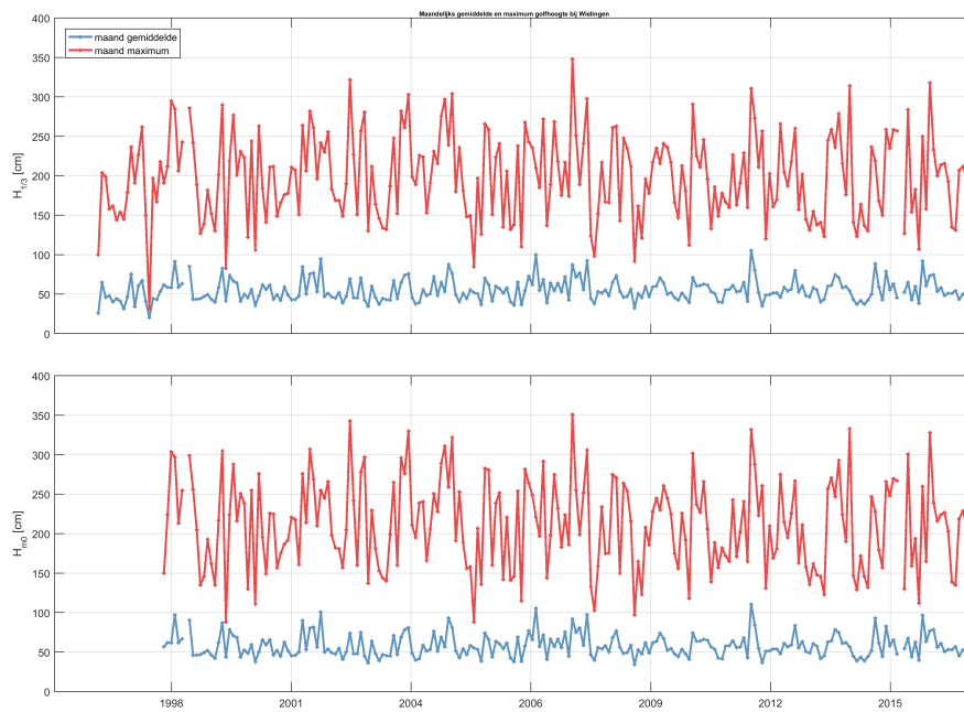
Figuur 2.33: Maandlijks gemiddelde en maximum van de significante golfhoogte H_{1/3} (boven) en H_{m0} (onder) voor station Wielingen.
