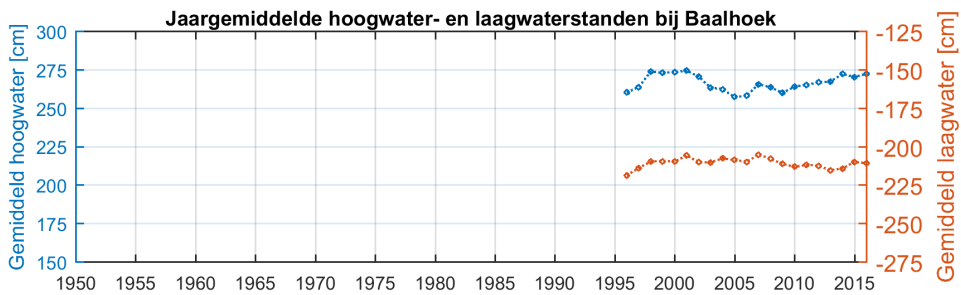
Figuur 2.14: Jaargemiddelde hoog- en laagwaterstanden bij Baalhoek
