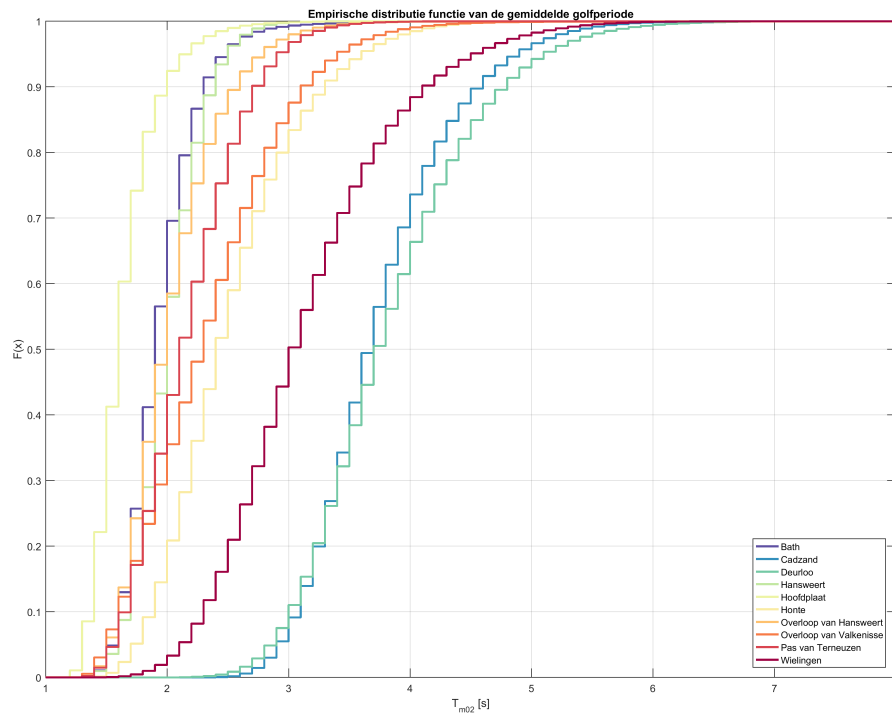
Figuur 2.41: Empirische distributiefunctie voor de significante golferiode berekend op basis van het spectrum voor alle beschikbare data tussen 1998 en 2015
