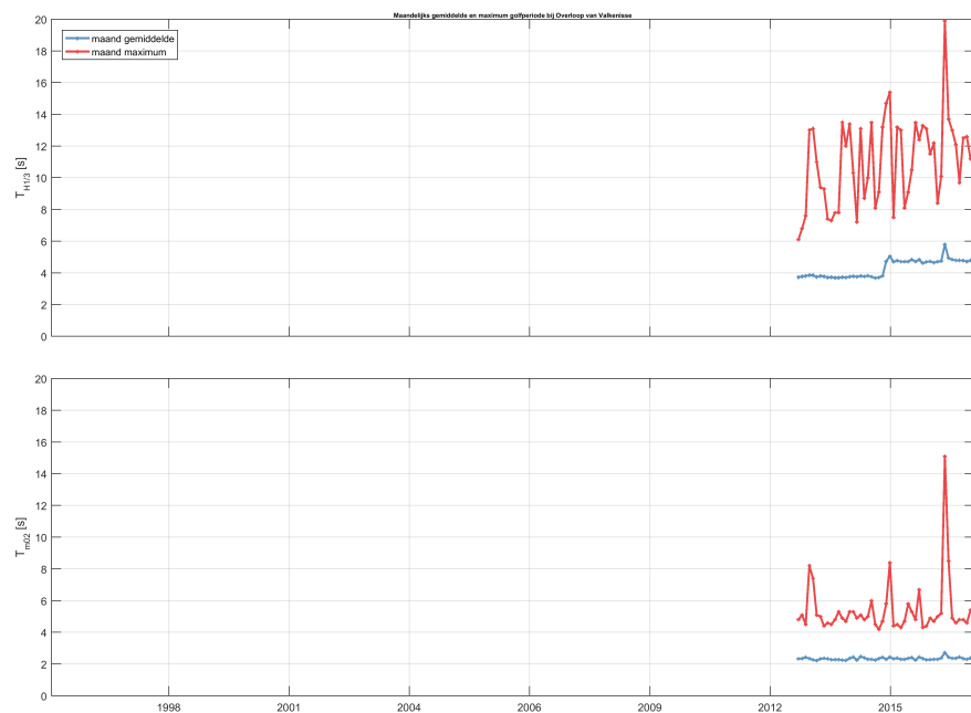
Figuur 2.49: Maandelijks gemiddelde en maximum van de golfperiode T_{H1/3} (boven) en T_{M02} (onder) voor station Overloop van Valkenisse.
