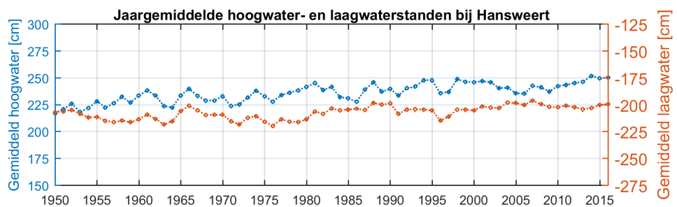
Figuur 2.12: Jaargemiddelde hoog- en laagwaterstanden bij Hansweert
