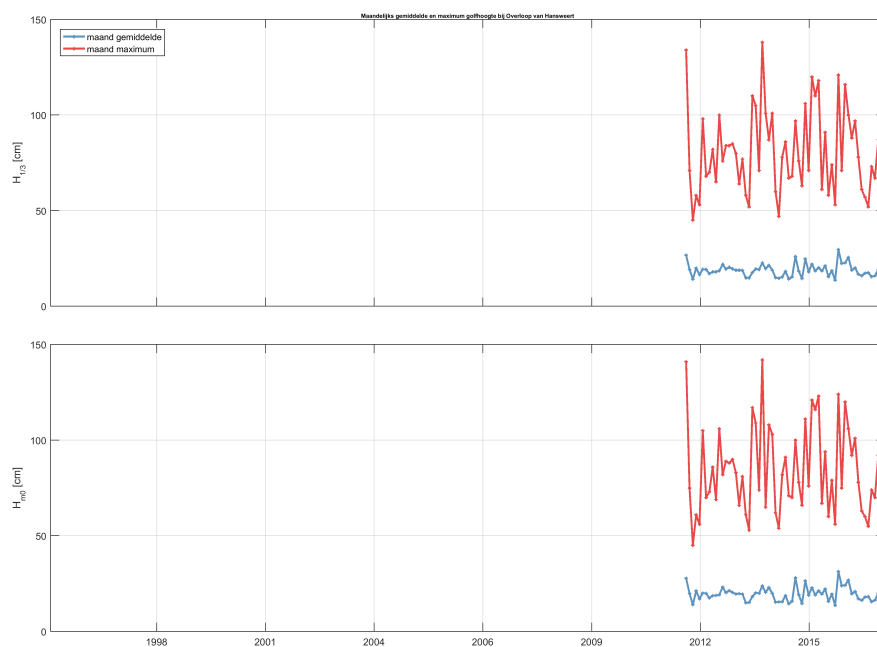
Figuur 2.36: Maandelijks gemiddelde en maximum van de significante golfhoogte H_{1/3} (boven) en H_{m0} (onder) voor station Overloop van Hansweert.
