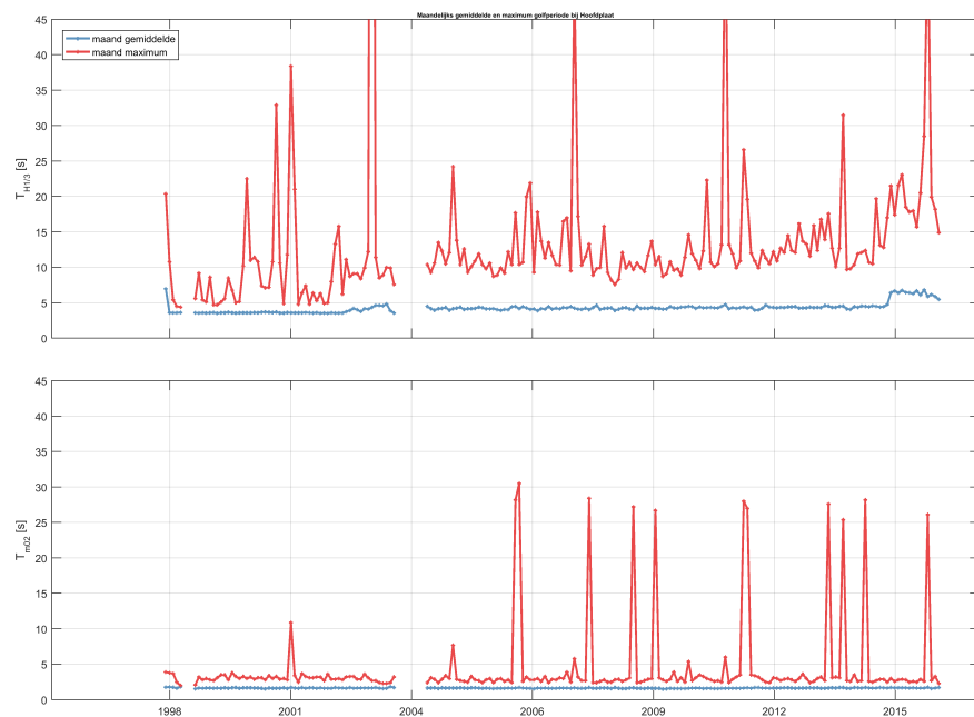
Figuur 2.45: Maandelijks gemiddelde en maximum van de golfperiode T_{H1/3} (boven) en T_{M02} (onder) voor station Hoofdplaat.
