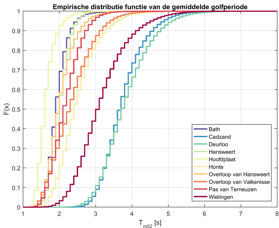
Figuur 2.40: Empirische distributiefunctie voor de significante golfperiode berekend op basis van het spectrum voor alle beschikbare data tussen 1998 en 2015
