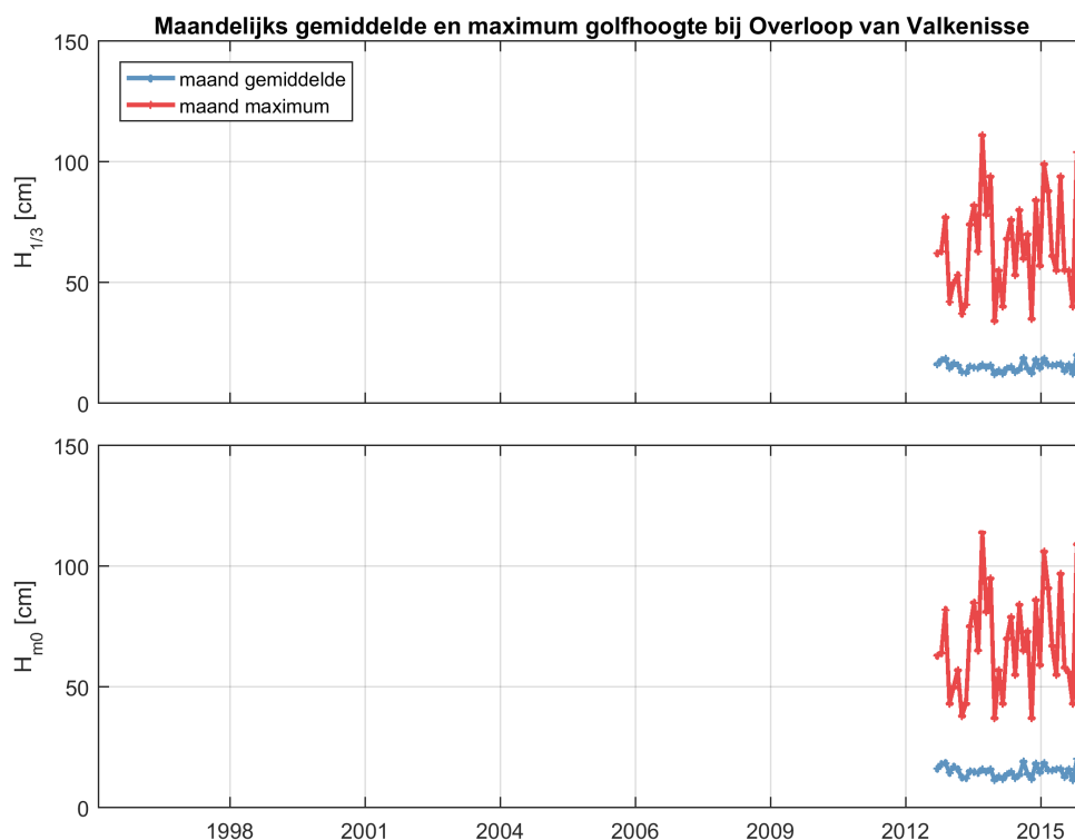
Figuur 2.37: Maandelijks gemiddelde en maximum van de significante golfhoogte H_{1/3} (boven) en H_{m0} (onder) voor station Overloop van Valkenisse.
