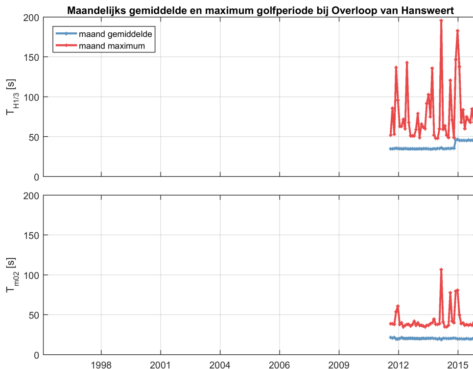
Figuur 2.46: Maandelijks gemiddelde en maximum van de golfperiode T_{H1/3} (boven) en T_{M02} (onder) voor station Overloop van Hansweert.
