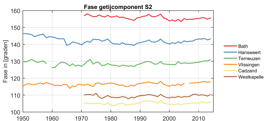
Figuur 2.25: Fase van de S2-getijcomponent voor de landelijke meetstations.
