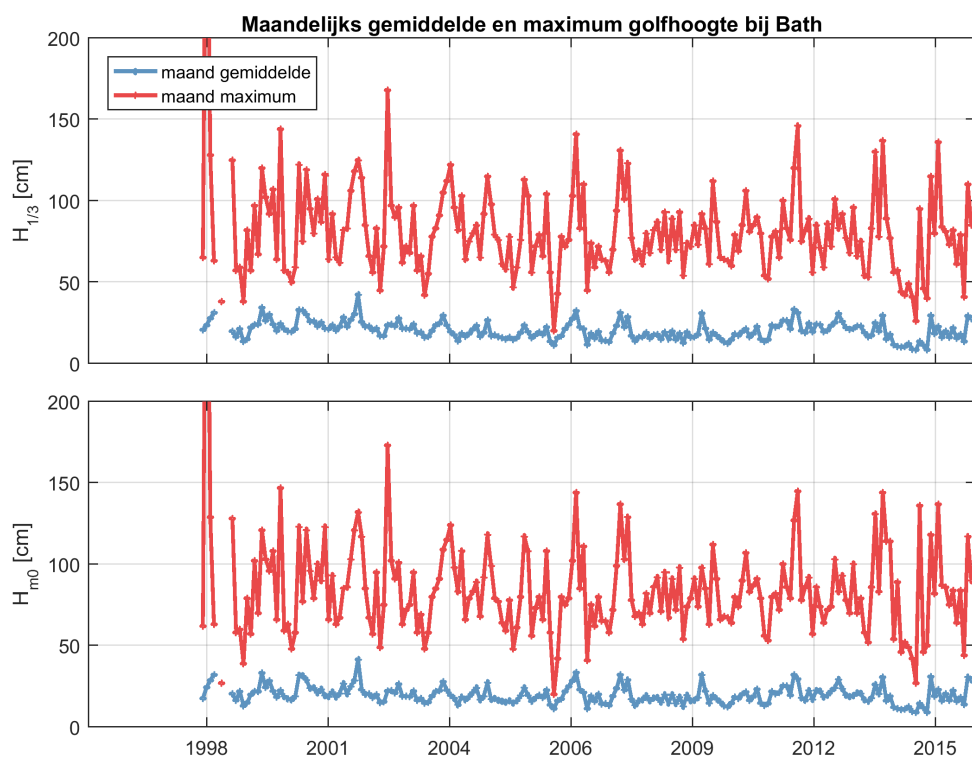
Figuur 2.38: Maandelijks gemiddelde en maximum van de significante golfhoogte H_{1/3} (boven) en H_{m0} (onder) voor station Bath.
