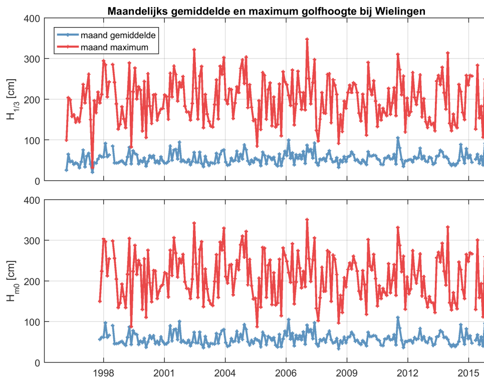
Figuur 2.32: Maandelijks gemiddelde en maximum van de significante golfhoogte H_{1/3} (boven) en H_{m0} (onder) voor station Wielingen.
