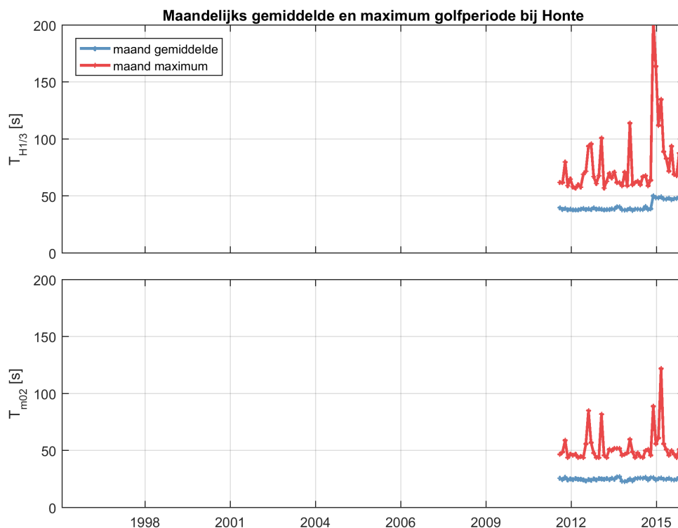
Figuur 2.45: Maandelijks gemiddelde en maximum van de golfperiode T_{H1/3} (boven) en T_{M02} (onder) voor station Honte.
