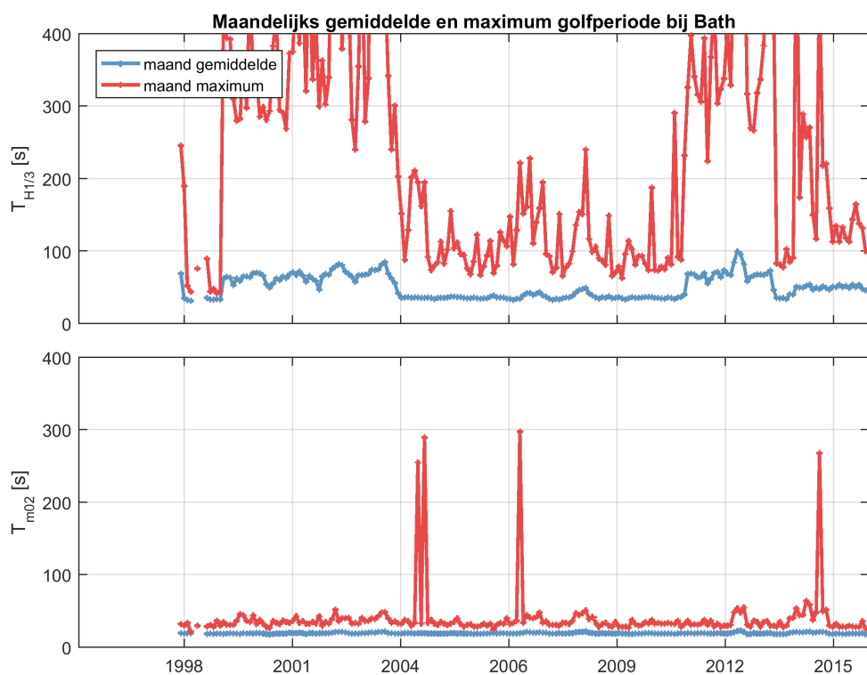
Figuur 2.49: Maandlijks gemiddelde en maximum van de golfperiode T_{H1/3} (boven) en T_{M02} (onder) voor station Bath.
