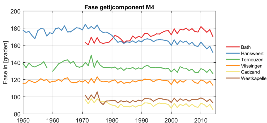
Figuur 2.24: Fase van de M4-getijcomponent voor de landelijke meetstations.
