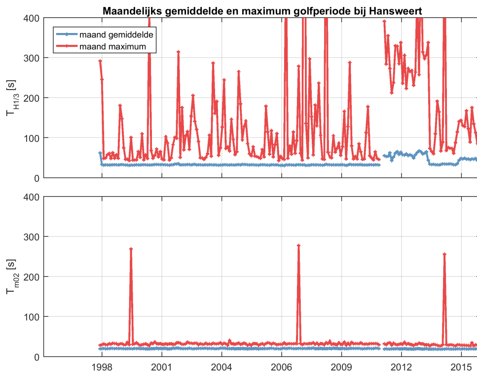
Figuur 2.47: Maandelijks gemiddelde en maximum van de golfperiode T_{H1/3} (boven) en T_{M02} (onder) voor station Hansweert.
