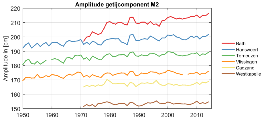
Figuur 2.20: Amplitude van de M2-getijcomponent voor de landelijke meetstations.
