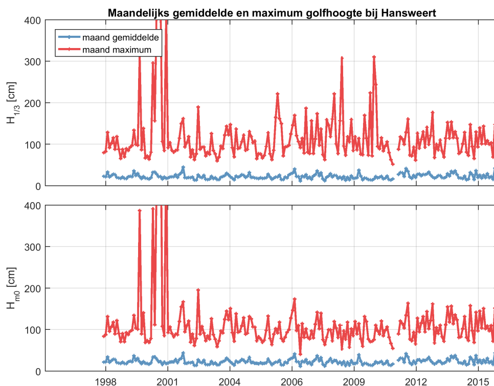
Figuur 2.36: Maandelijks gemiddelde en maximum van de significante golfhoogte H_{1/3} (boven) en H_{m0} (onder) voor station Hansweert.
