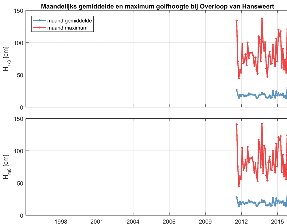
Figuur 2.35: Maandelijks gemiddelde en maximum van de significante golfhoogte H_{1/3} (boven) en H_{m0} (onder) voor station Overloop van Hansweert.
