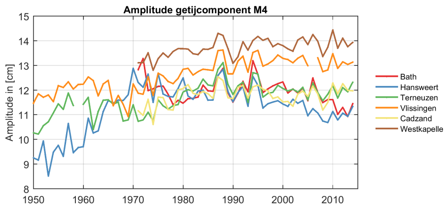
Figuur 2.21: Amplitude van de M4-getijcomponent voor de landelijke meetstations.
