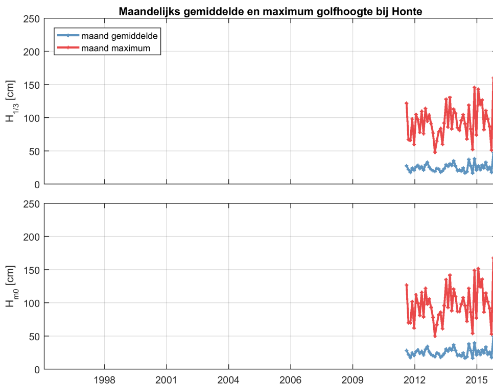
Figuur 2.34: Maandelijks gemiddelde en maximum van de significante golfhoogte H_{1/3} (boven) en H_{m0} (onder) voor station Honte.
