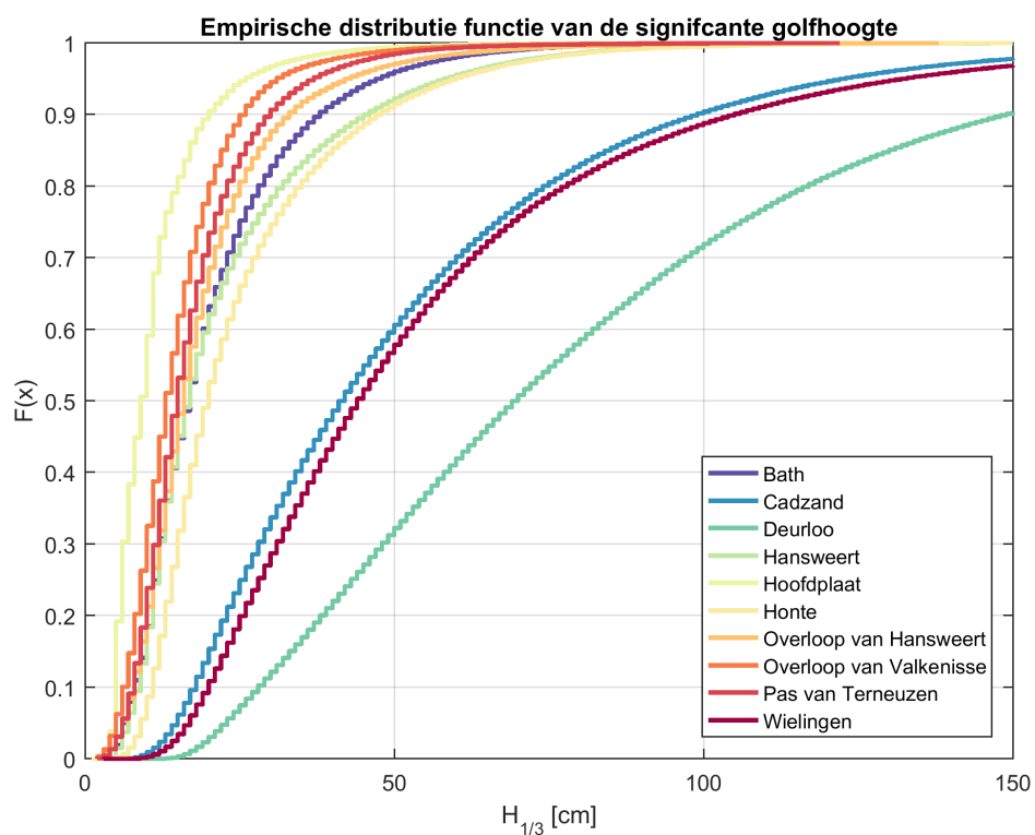
Figuur 2.29: Empirische distributiefunctie voor de significante golfhoogte berekend op basis van het spectrum voor alle beschikbare data tussen 1998 en 2015
