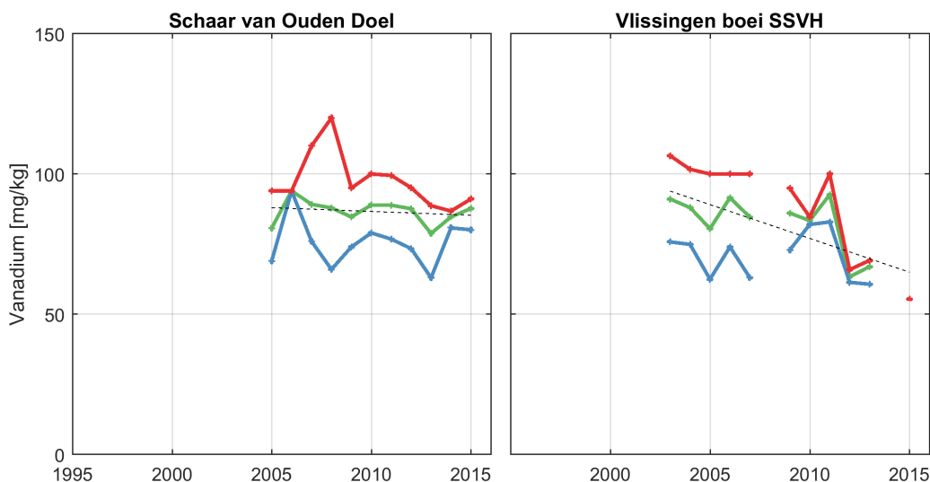
Figuur 4.11: Jaarlijks gemiddelde (groen), minimum (blauw) en maximum (rood) van de Vanadium voor alle stations
