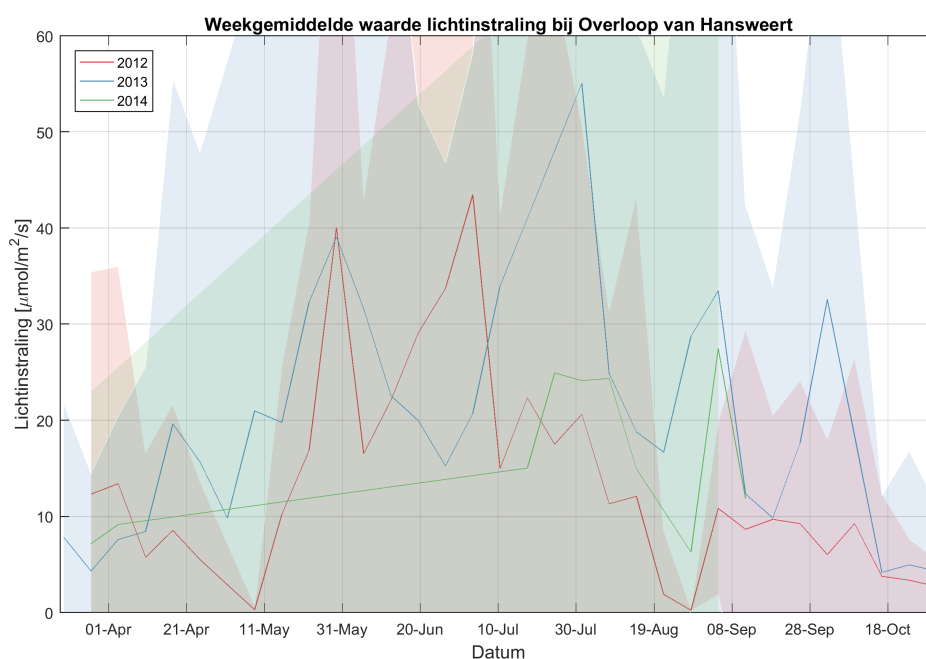
Figuur 3.101: Weekgemiddelde waarden van de lichtinstraling zoals gemeten tijdens de continue metingen van 2012, 2013 en 2014 bij station Overloop van Hansweert. De band rondom de gemiddelden waarde is de onzekerheid gegeven door de standaard deviatie.
