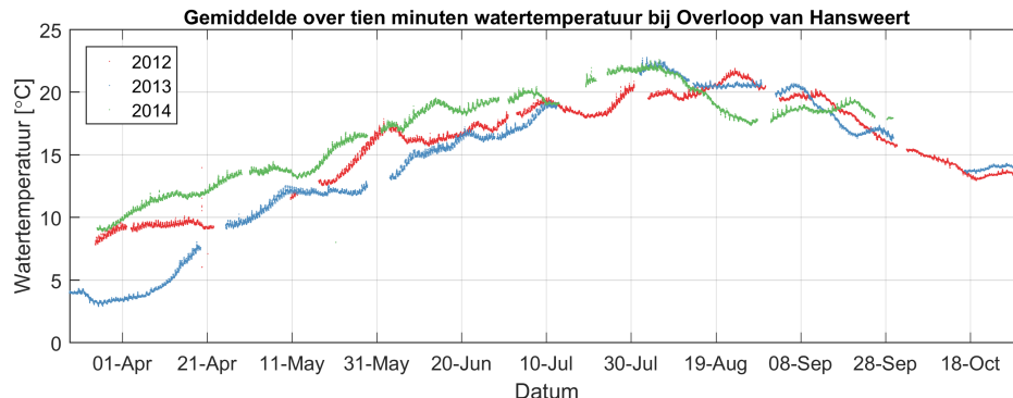
Figuur 3.90: Tijdsree van de watertemperatuur zoals gemeten tijdens de continue metingen van 2012, 2013 en 2014 bij station Overloop van Hansweert.
