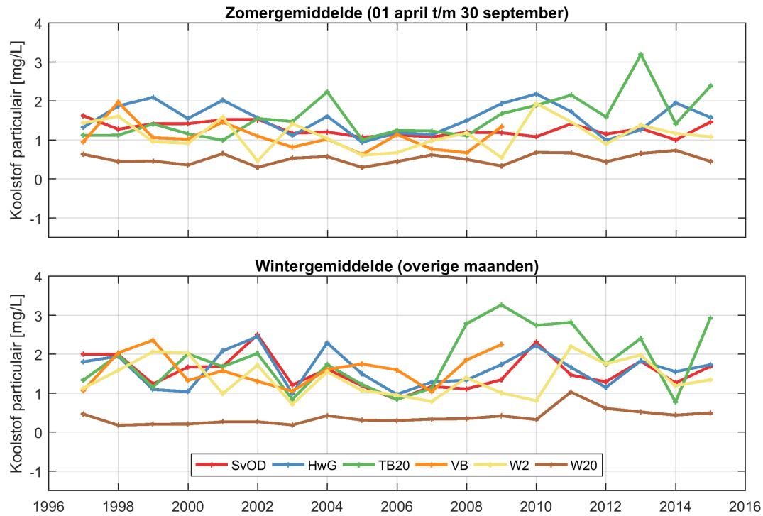
Figuur 3.53: Gemiddeld waarden voor de hoeveelheid particuliere koolstofgehalte gedurende de zomer en de winter in het oppervlaktewater van de Westerschelde en de monding
