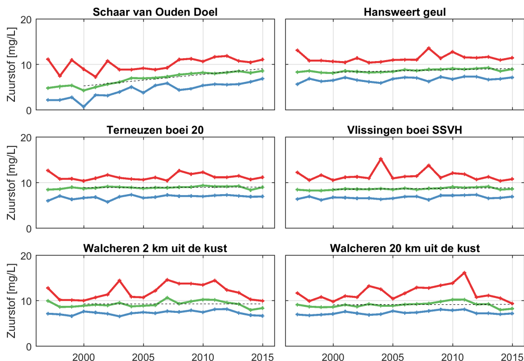
Figuur 3.12: Jaarlijks gemiddelde, minimum en maximum van het zuurstofgehalte in mg/L in het oppervlaktewater van de Westerschelde en de monding
