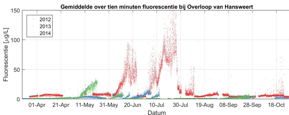
Figuur 3.102: Tijdsreef van de fluorescentie zoals gemeten tijdens de continue metingen van 2012, 2013 en 2014 bij station Overloop van Hansweert.
