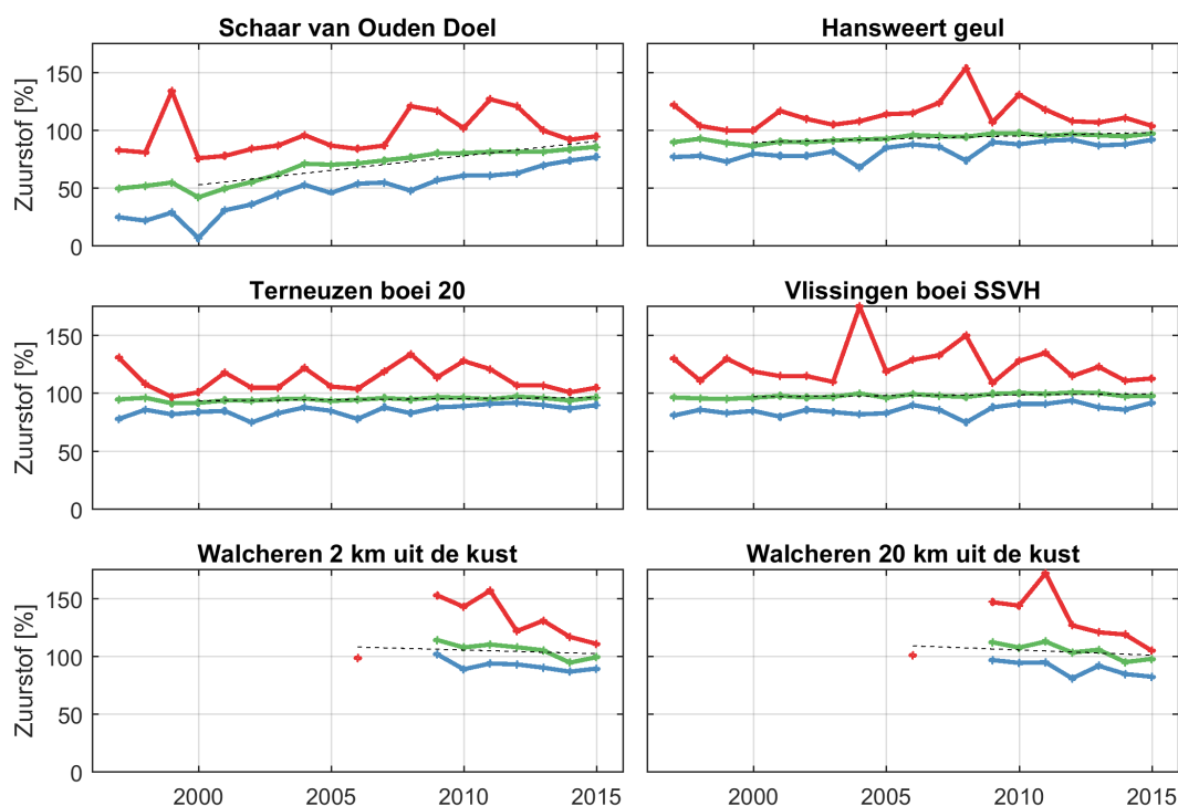
Figuur 3.11: Jaarlijks gemiddelde, minimum en maximum van het zuurstofverzadigingspercentage in het oppervlaktewater van de Westerschelde en de monding
