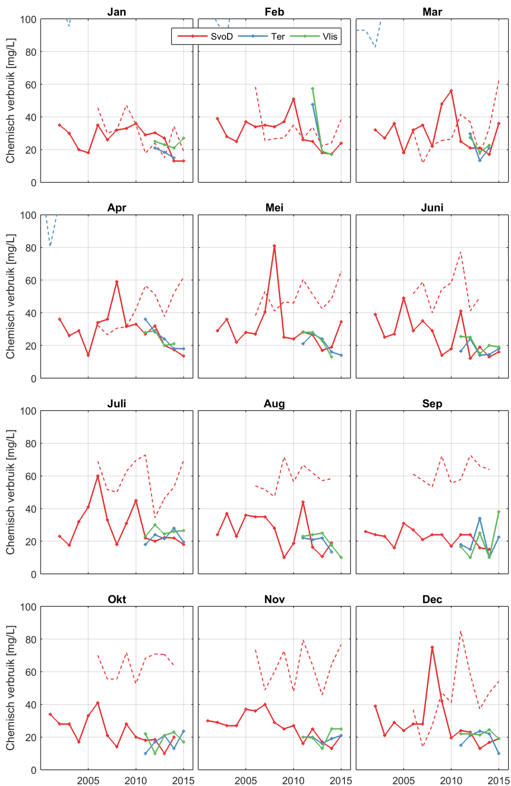
Figuur 3.23: Maandgemiddelde waarde van het chemisch zuurstofverbruik in het oppervlaktewater van de Westerschelde en de monding. De stippellijn geeft de bepalingsgrens weer.
