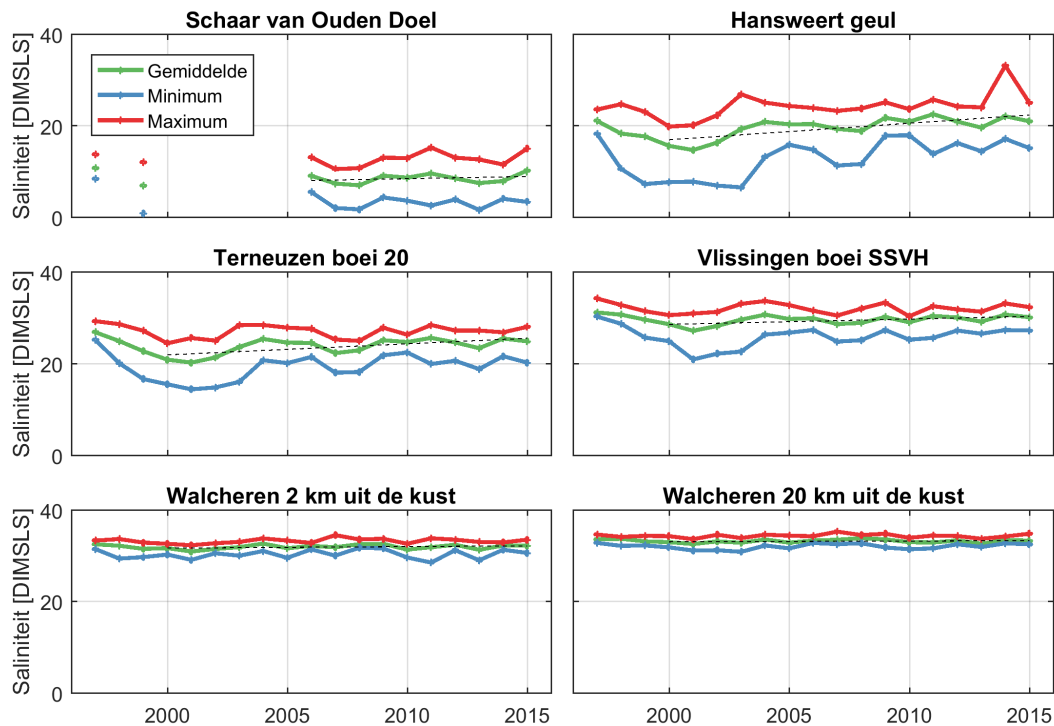
Figuur 3.2: Jaarlijks gemiddelde, minimum en maximum van de saliniteit in de Westerschelde en in de monding.
