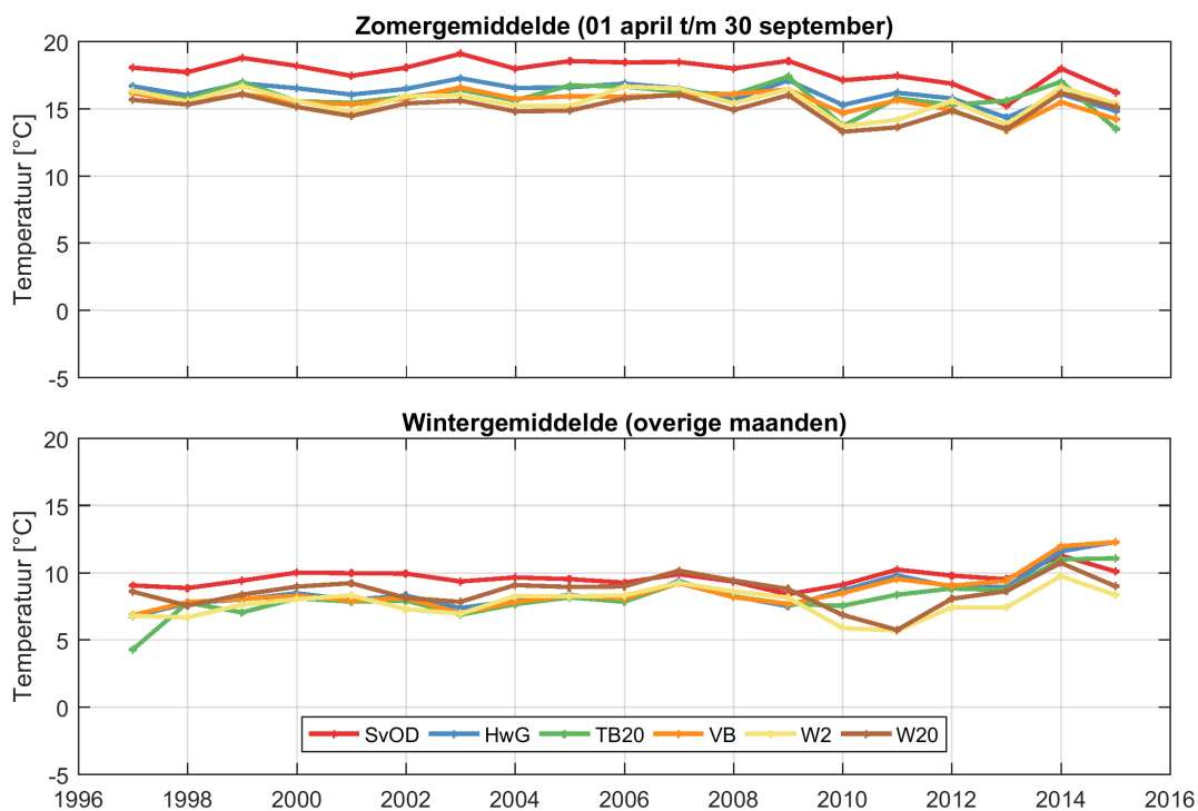
Figuur 3.6: Gemiddelde temperatuur gedurende de zomer en de winter in het oppervlaktewater van de Westerschelde en de monding.
