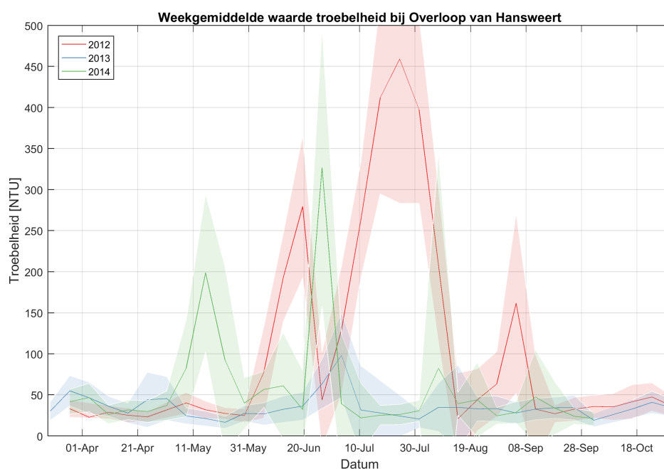
Figuur 3.98: Weekgemiddelde waarden van de troebelheid zoals gemeten tijdens de continue metingen van 2012, 2013 en 2014 bij station Overloop van Hansweert. De band rondom de gemiddelden waarde is de onzekerheid gegeven door de standaard deviatie.
