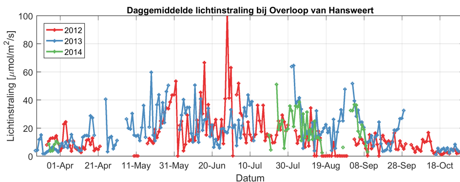
Figuur 3.100: Daggemiddelde waardes van de lichtinstraling zoals gemeten tijdens de continue metingen van 2012, 2013 en 2014 bij station Overloop van Hansweert.
