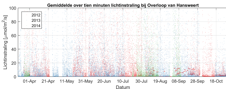
Figuur 3.99: Tijdsreeks van de lichtinstraling zoals gemeten tijdens de continue metingen van 2012, 2013 en 2014 bij station Overloop van Hansweert.
