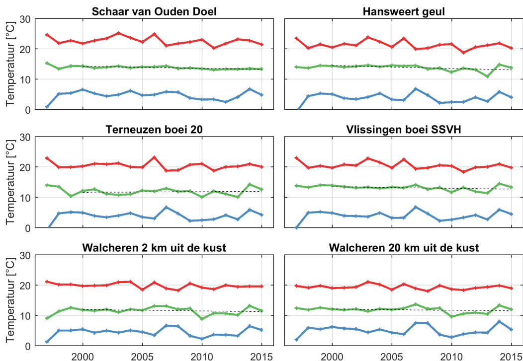
Figuur 3.5: Jaarlijks gemiddelde (groen), minimum (blauw) en maximum (rood) van de temperatuur in de Westerschelde en in de monding
