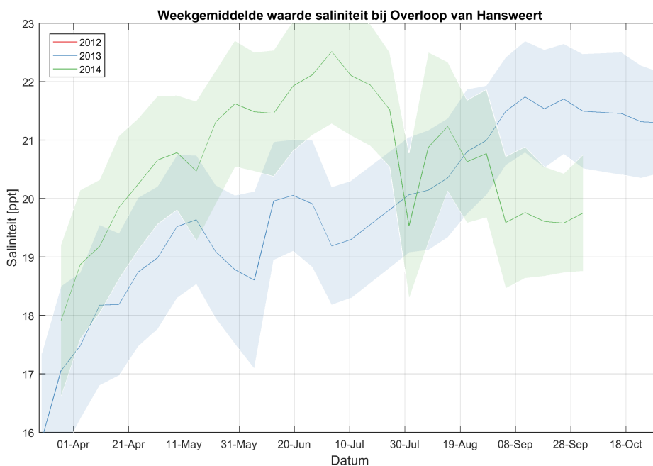
Figuur 3.89: Weekgemiddelde waarden van de saliniteit zoals gemeten tijdens de continue metingen van 2012, 2013 en 2014 bij station Overloop van Hansweert. De band rondom de gemiddelden waarde is de onzekerheid gegeven door de standaard deviatie.
