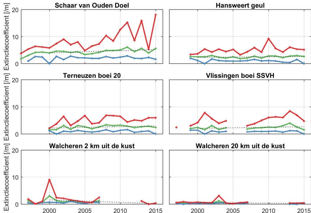
Figuur 3.27: Jaarlijks gemiddelde, minimum en maximum van de extinctiecoëfficiënt in het oppervlaktewater van de Westerschelde en de monding.
