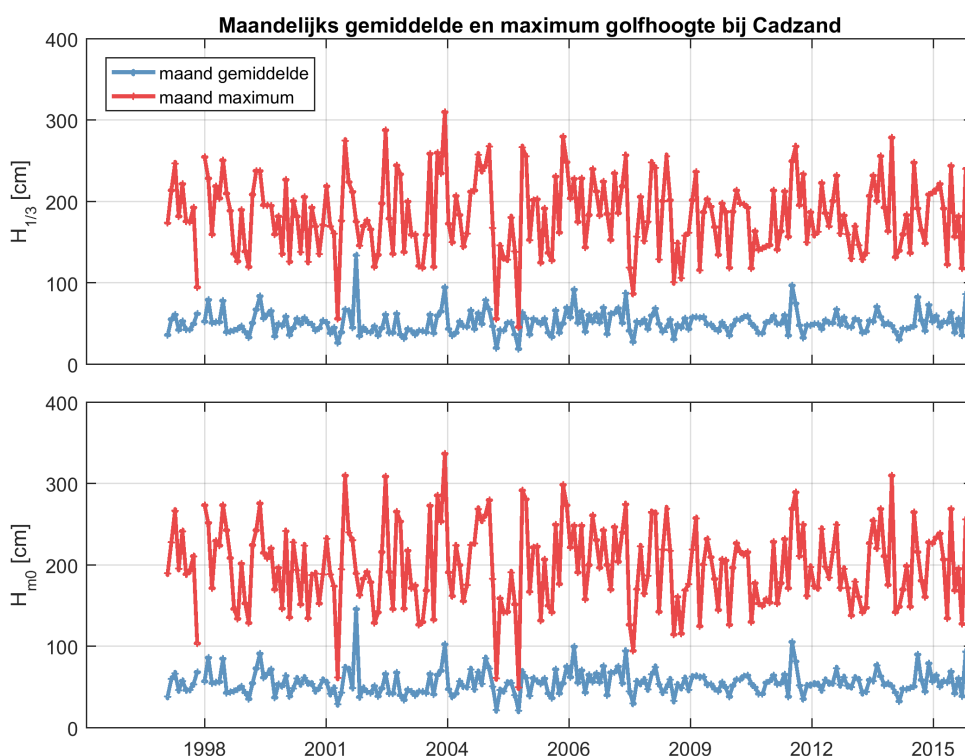
Figuur 2.31: Maandelijks gemiddelde en maximum van de significante golfhoogte H_{1/3} (boven) en H_{m0} (onder) voor station Cadzand.
