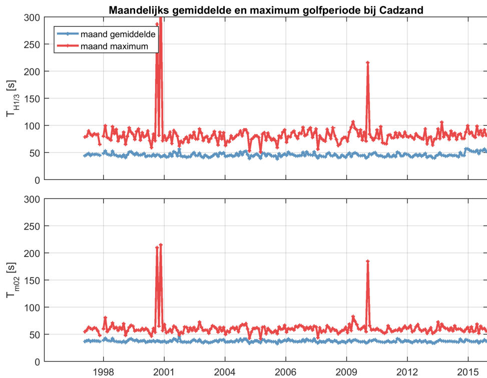
Figuur 2.42: Maandelijks gemiddelde en maximum van de golfperiode T_{H1/3} (boven) en T_{M02} (onder) voor station Cadzand.
