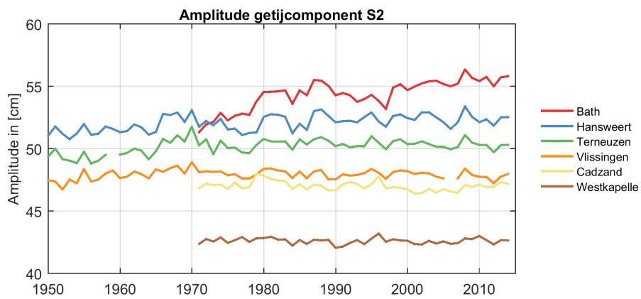
Figuur 2.22: Amplitude van de S2-getijcomponent voor de landelijke meetstations.
