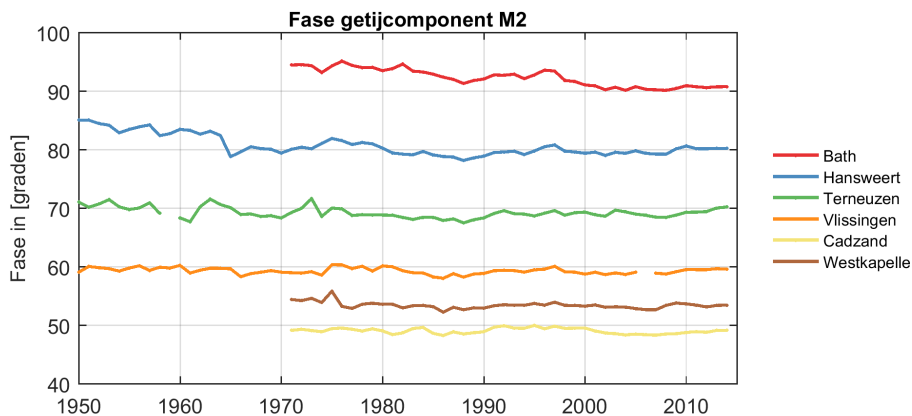
Figuur 2.23: Fase van de M2-getijcomponent voor de landelijke meetstations.
