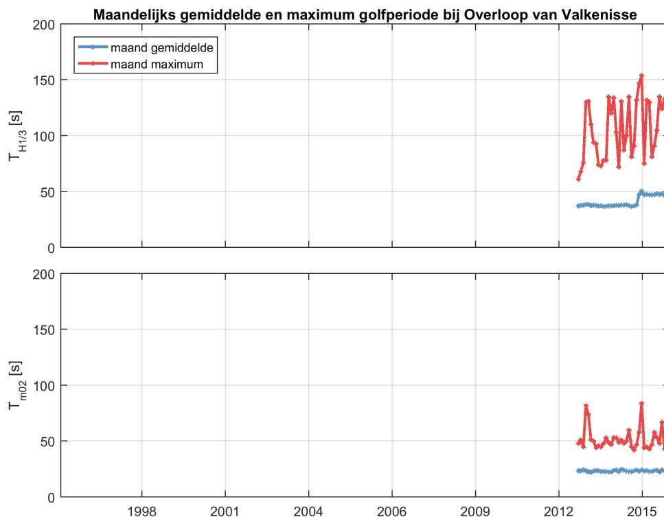
Figuur 2.48: Maandelijks gemiddelde en maximum van de golfperiode T_{H1/3} (boven) en T_{M02} (onder) voor station Overloop van Valkenisse.
