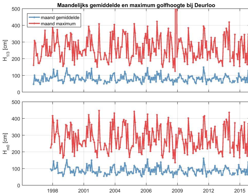
Figuur 2.30: Maandelijks gemiddelde en maximum van de significante golfhoogte H_{1/3} (boven) en H_{m0} (onder) voor station Deurloo.
