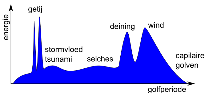
Figuur 2.26: Voorbeeld van een geschematiseerd golfspectrum op zee (naar: www.infrawiki.nl )
