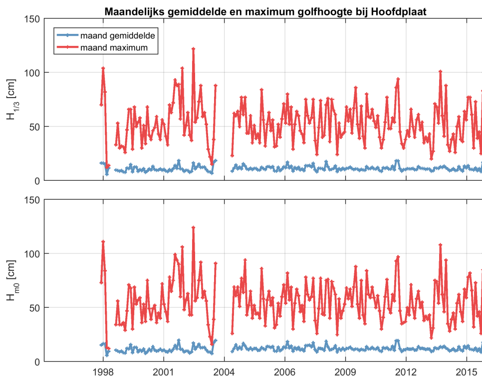
Figuur 2.33: Maandelijks gemiddelde en maximum van de significante golfhoogte H_{1/3} (boven) en H_{m0} (onder) voor station Hoofdplaat.
