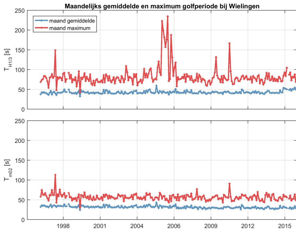
Figuur 2.43: Maandelijks gemiddelde en maximum van de golfperiode T_{H1/3} (boven) en T_{M02} (onder) voor station Wielingen.
