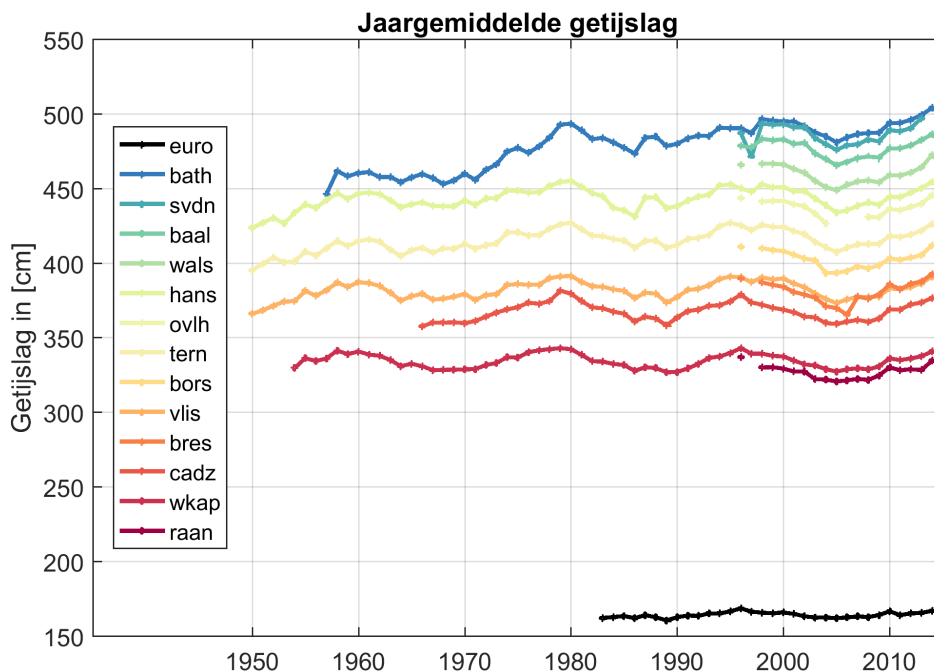
Figuur 2.18: De gemiddelde getijslag over tijd op de Noordzee, in de monding en in de Westerschelde
