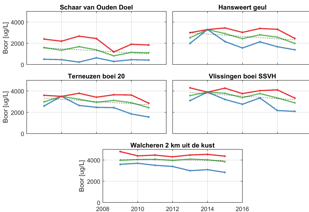
Figuur 3.62: Jaarlijks gemiddelde, minimum en maximum van het totale boorgehalte in het oppervlaktewater van de Westerschelde en de monding.
