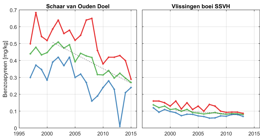
Figuur 4.14: Jaarlijks gemiddelde (groen), minimum (blauw) en maximum (rood) van de benzoapyreen voor alle stations
