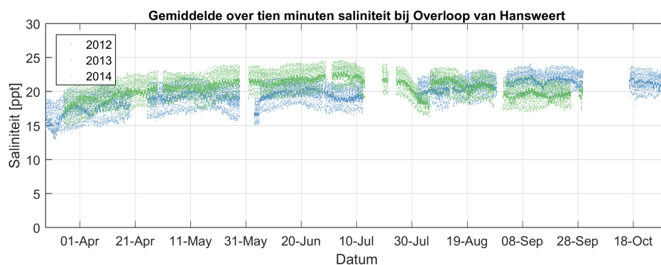
Figuur 3.87: Tijdsreef van de saliniteit zoals gemeten tijdens de continue metingen van 2012, 2013 en 2014 bij station Overloop van Hansweert.
