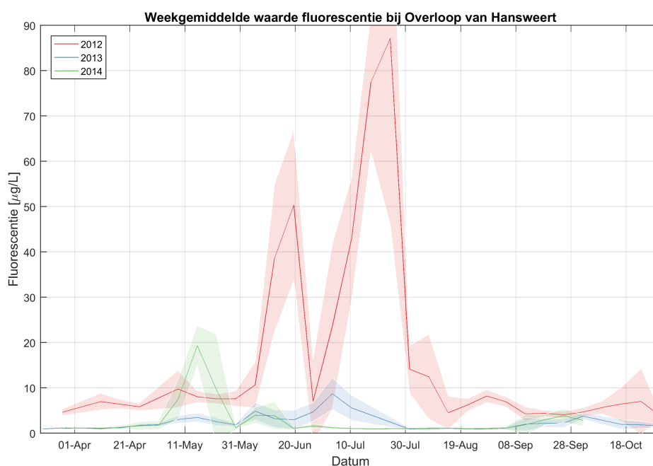
Figuur 3.104: Weekgemiddelde waarden van de fluorescentie zoals gemeten tijdens de continue metingen van 2012, 2013 en 2014 bij station Overloop van Hansweert. De band rondom de gemiddelden waarde is de onzekerheid gegeven door de standaard deviatie.
