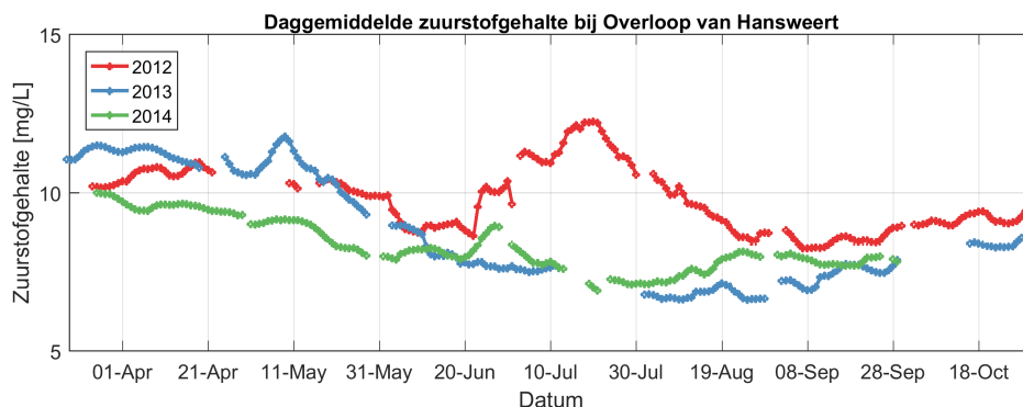
Figuur 3.94: Daggemiddelde waarden van het zuurstofgehalte zoals gemeten tijdens de continue metingen van 2012, 2013 en 2014 bij station Overloop van Hansweert.
