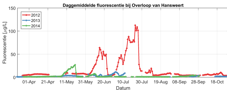
Figuur 3.103: Daggemiddelde waardes van de fluorescentie zoals gemeten tijdens de continue metingen van 2012, 2013 en 2014 bij station Overloop van Hansweert.
