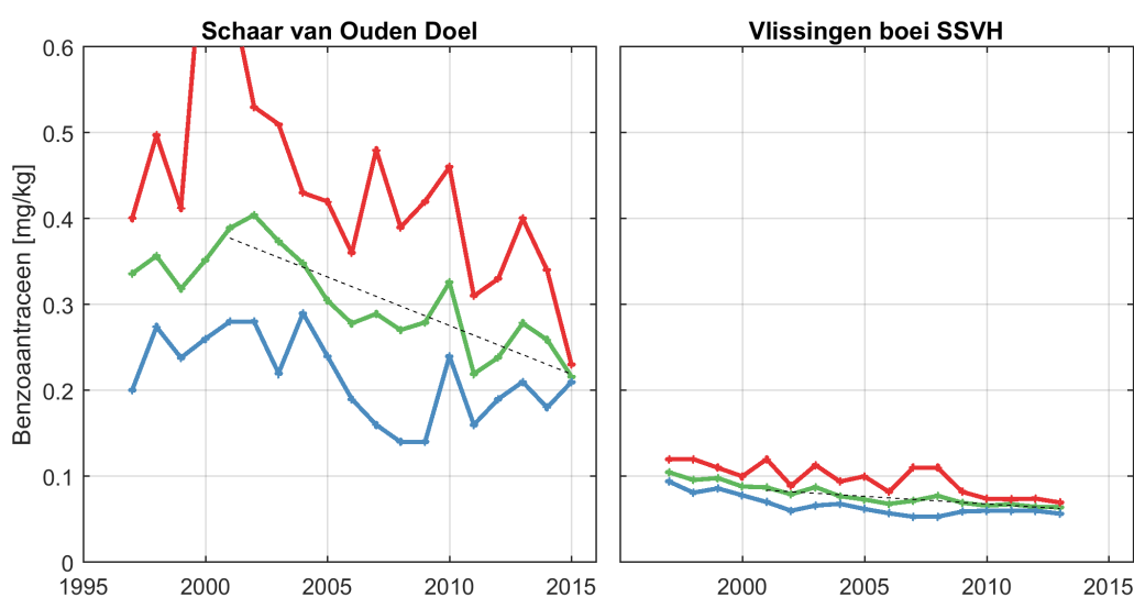
Figuur 4.16: Jaarlijks gemiddelde (groen), minimum (blauw) en maximum (rood) van de benzoaantraceneen voor alle stations
