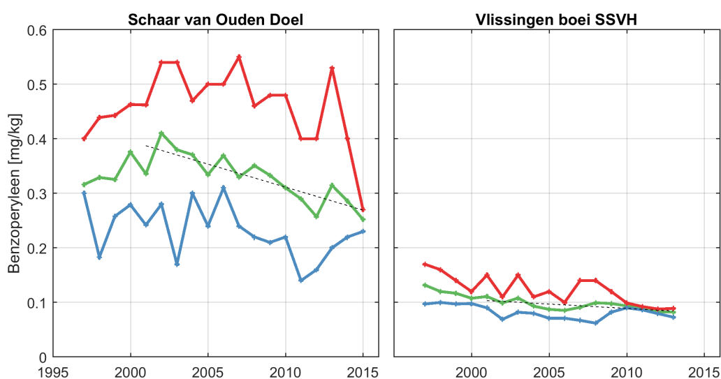
Figuur 4.15: Jaarlijks gemiddelde (groen), minimum (blauw) en maximum (rood) van de benzoperyleen voor alle stations
