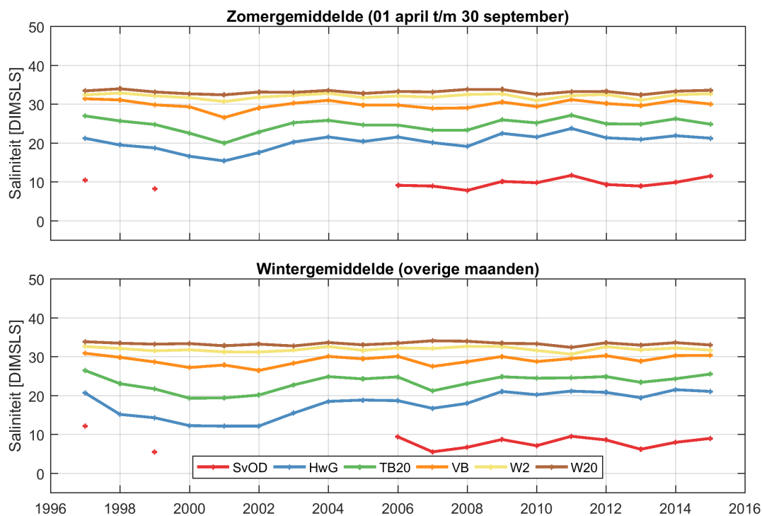
Figuur 3.3: Gemiddelde saliniteit gedurende de zomer en de winter in het oppervlaktewater van de Westerschelde en de monding.
