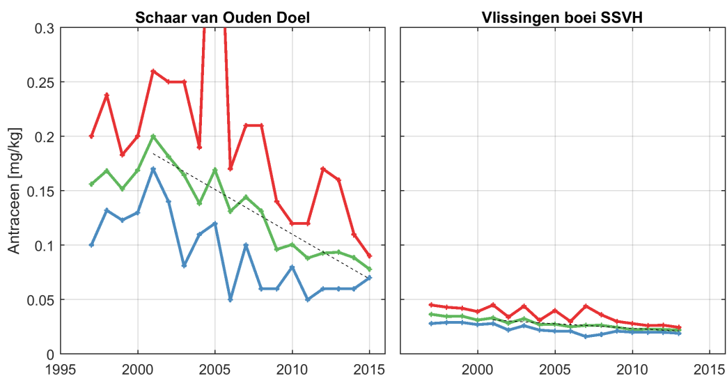
Figuur 4.13: Jaarlijks gemiddelde (groen), minimum (blauw) en maximum (rood) van de antraceen voor alle stations
