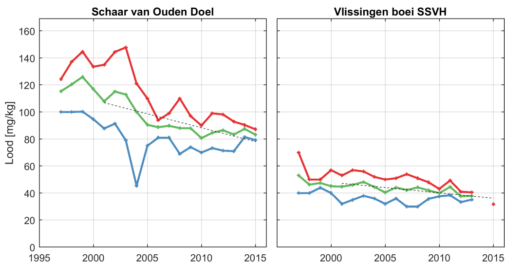
Figuur 4.10: Jaarlijks gemiddelde (groen), minimum (blauw) en maximum (rood) van de lood voor alle stations
