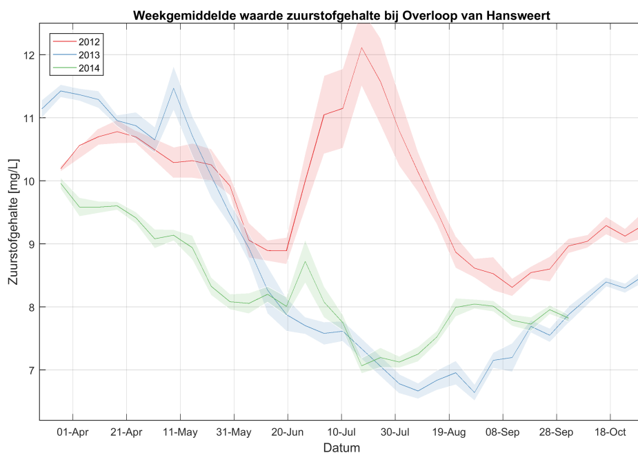
Figuur 3.95: Weekgemiddelde waarden van het zuurstofgehalte zoals gemeten tijdens de continue metingen van 2012, 2013 en 2014 bij station Overloop van Hansweert. De band rondom de gemiddelden waarde is de onzekerheid gegeven door de standaard deviatie.
