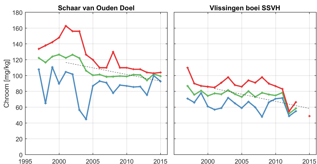
Figuur 4.6: Jaarlijks gemiddelde (groen), minimum (blauw) en maximum (rood) van de chroom voor alle stations
