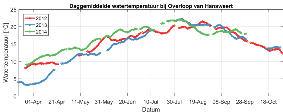
Figuur 3.91: Daggemiddelde waarden van de watertemperatuur zoals gemeten tijdens de continue metingen van 2012, 2013 en 2014 bij station Overloop van Hansweert.. De band rondom de gemiddelden waarde is de onzekerheid gegeven door de standaard deviatie.
