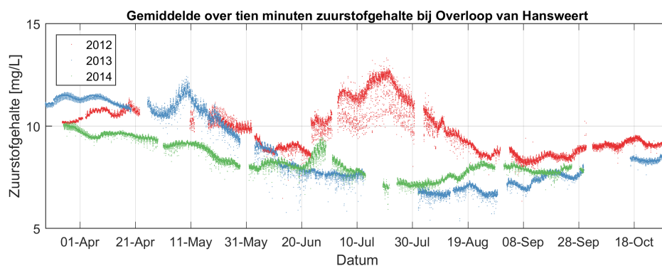
Figuur 3.93: Tijdserie van het zuurstofgehalte zoals gemeten tijdens de continue metingen van 2012, 2013 en 2014 bij station Overloop van Hansweert.
