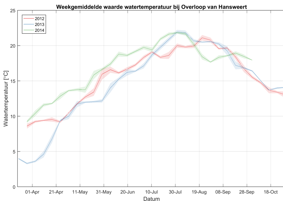
Figuur 3.92: Weekgemiddelde waarden van de watertemperatuur zoals gemeten tijdens de continue metingen van 2012, 2013 en 2014 bij station Overloop van Hansweert. De band rondom de gemiddelden waarde is de onzekerheid gegeven door de standaard deviatie.
