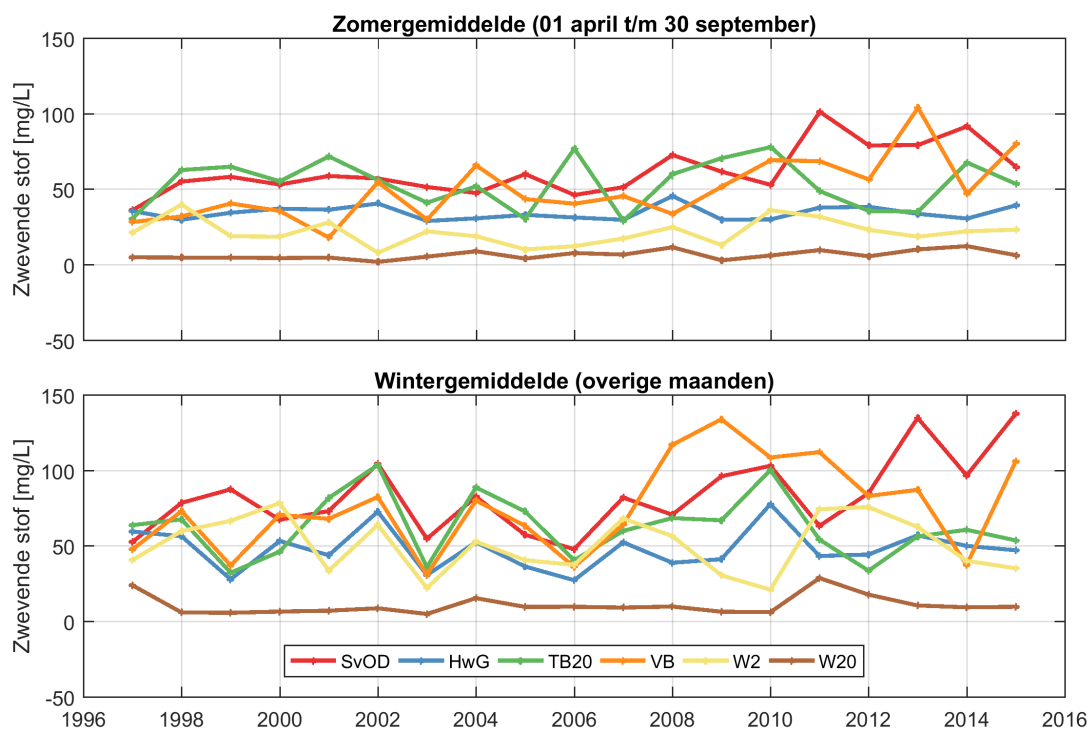
Figuur 3.32: Gemiddeld waarden voor de hoeveelheid zwevende stof gedurende de zomer en de winter in het oppervlaktewater van de Westerschelde en de monding
