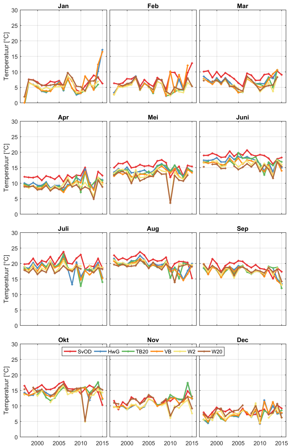
Figuur 3.7: Maandgemiddelde temperatuur in het oppervlaktewater van de Westerschelde en de monding.
