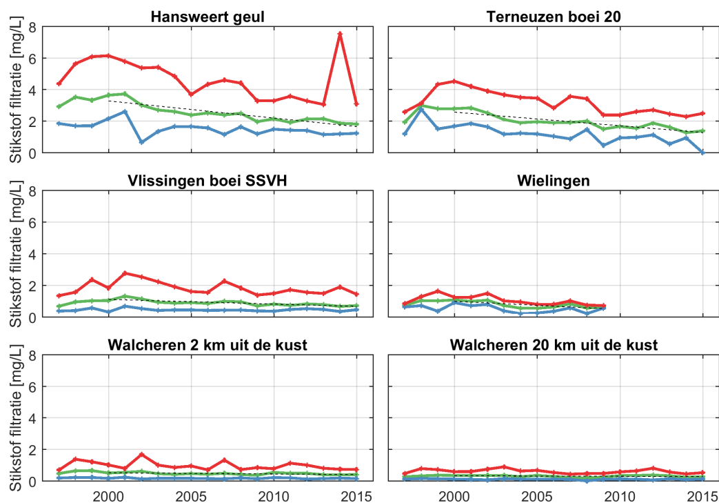
Figuur 3.33: Jaarlijks gemiddelde, minimum en maximum van het stikstofgehalte in het oppervlaktewater van de Westerschelde en de monding.
