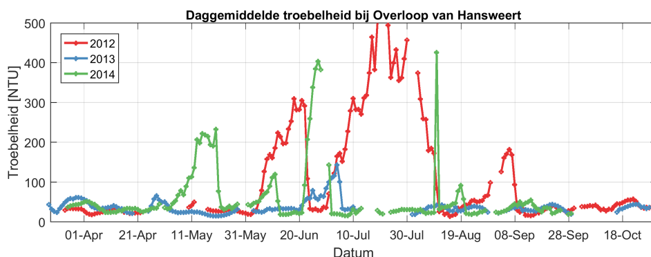
Figuur 3.97: Daggemiddelde waarden van de troebelheid zoals gemeten tijdens de continue metingen van 2012, 2013 en 2014 bij station Overloop van Hansweert.
