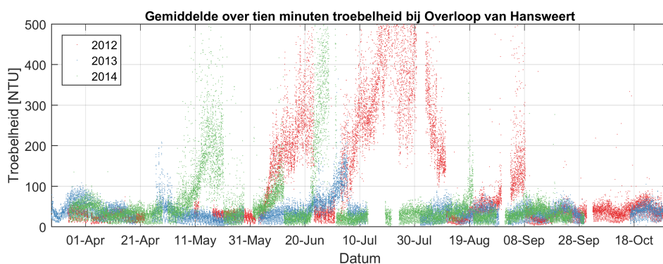
Figuur 3.96: Tijdsree van de troebelheid zoals gemeten tijdens de continue metingen van 2012, 2013 en 2014 bij station Overloop van Hansweert.
