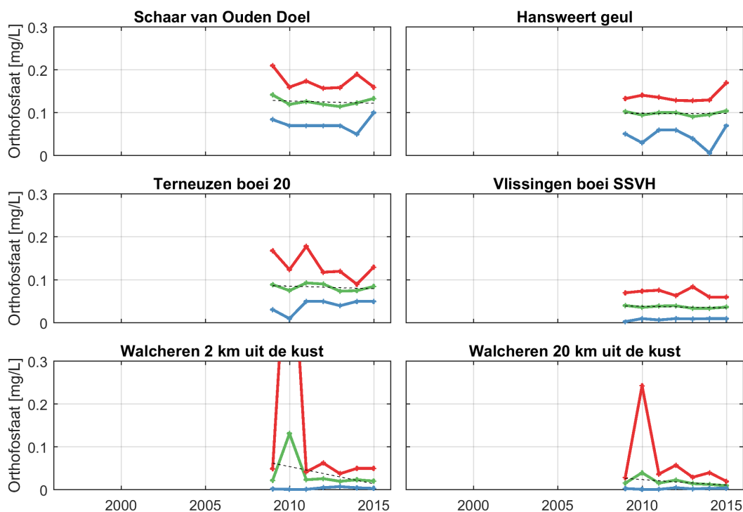
Figuur 3.42: Jaarlijks gemiddelde, minimum en maximum van het orthofosfaatgehalte in mg/L in het oppervlaktewater van de Westerschelde en de monding.
