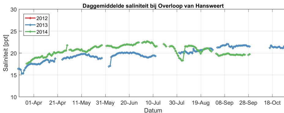
Figuur 3.88: Daggemiddelde waarden van de saliniteit zoals gemeten tijdens de continue metingen van 2012, 2013 en 2014 bij station Overloop van Hansweert.
