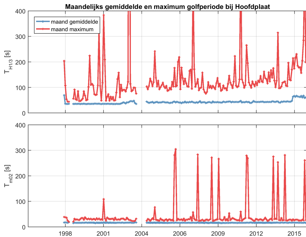
Figuur 2.44: Maandelijks gemiddelde en maximum van de golfperiode T_{H1/3} (boven) en T_{M02} (onder) voor station Hoofdplaat.
