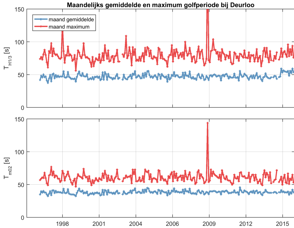
Figuur 2.41: Maandelijks gemiddelde en maximum van de golfperiode T_{H1/3} (boven) en T_{M02} (onder) voor station Deurloo.
