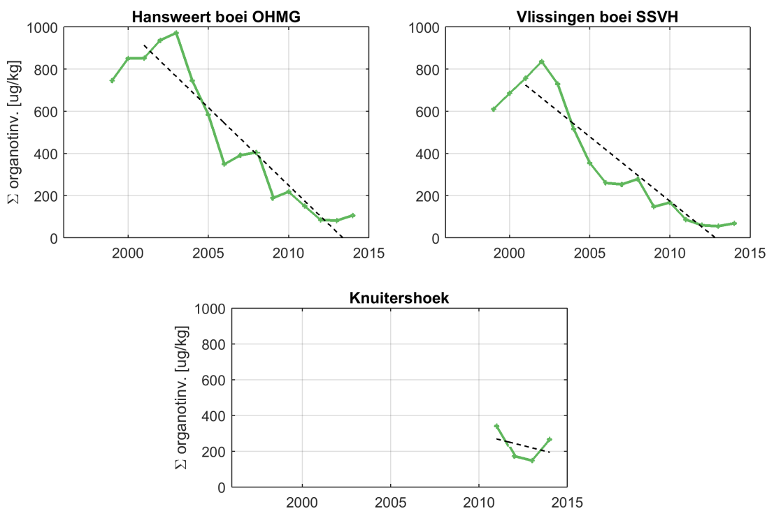
Figuur 5.18: Jaarlijks gesommeerde waarde van de organotinverbindingen in mossel voor 3 stations in de Westerschelde. Waarden zijn gepresenteerd in drooggewicht ( \mu\text{g}/\text{kg} ).
