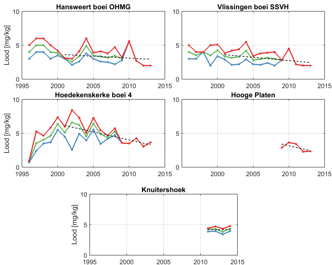
Figuur 5.11: Jaarlijks gemiddelde (groen), minimum (blauw) en maximum (rood) voor lood in mosselen (nat en droog) voor meerdere stations. Waardes zijn in drooggewicht gepresenteerd.
