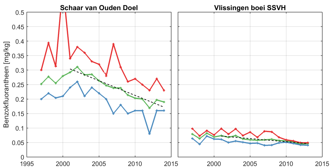
Figuur 4.17: Jaarlijks gemiddelde (groen), minimum (blauw) en maximum (rood) van de benzokfluorantheen voor alle stations
