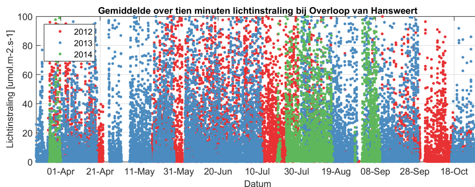
Figuur 3.68: Tijdserie van de lichtinstraling zoals gemeten tijdens de continue metingen van 2012, 2013 en 2014 bij station Overloop van Hansweert.
