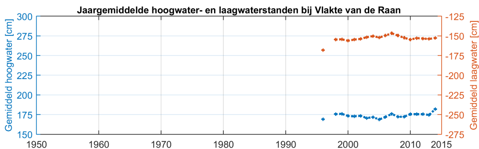
Figuur 2.4: Jaargemiddelde hoog- en laagwaterstanden bij de Vlakte van de Raan
