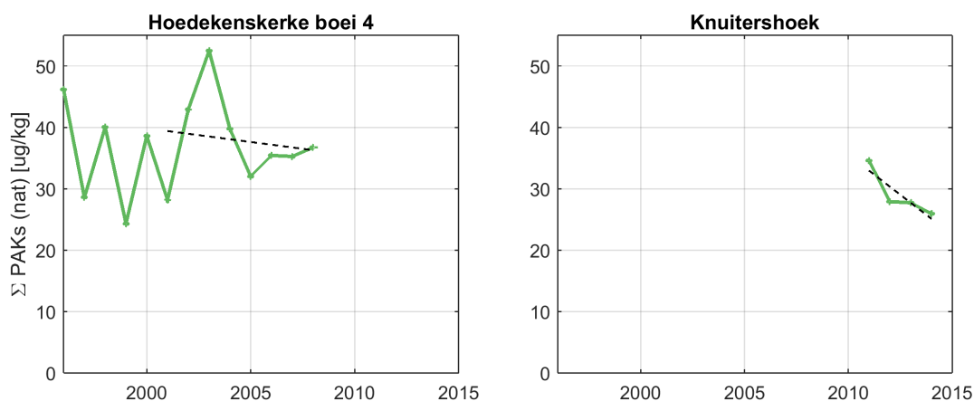
Figuur 5.14: Jaarlijks gesommeerde waarde van de 6 PAKs van Borneff in mossel bij Hoedekenskerke boei 4 en Knuitershoek. Waarden zijn in natgewicht gepresenteerd.
